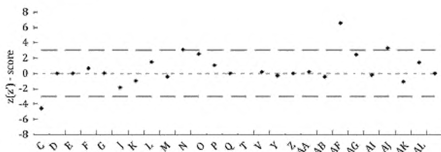
Рисунок A.1 – График Z-оценки измерения потерь сухой массы в процентах
