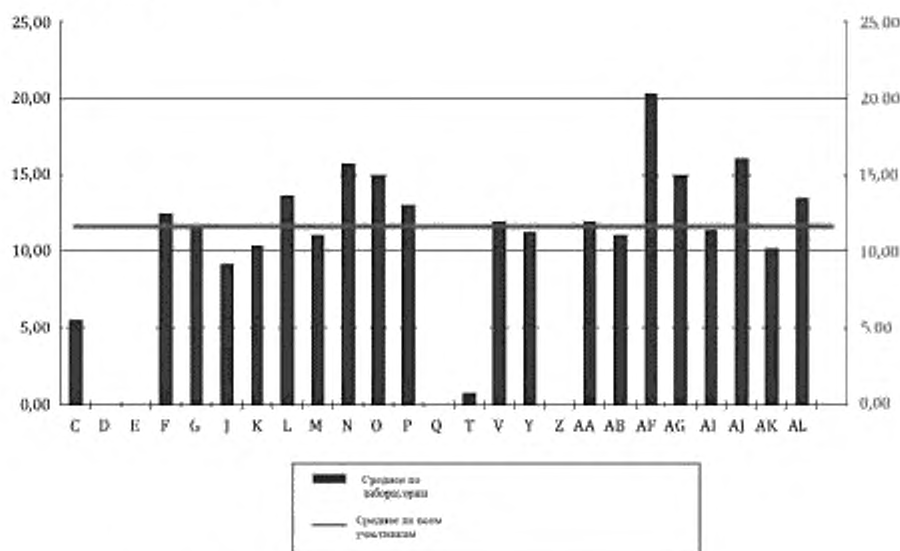
Рисунок A.2 – Гистограмма распределения потери сухой массы в процентах
