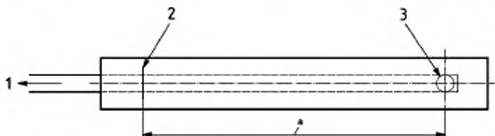
а — 2,50 м или менее, в зависимости от требуемой длины пробы 1 — натяжение; 2 — лезвие резака; 3 — направляющий стержень
