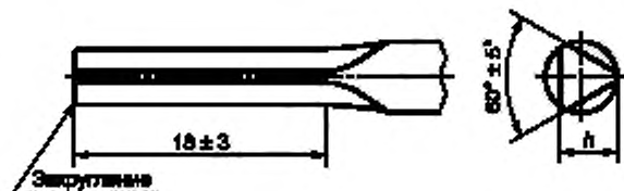
Рисунок 5 — Форма С (конец треугольного сечения)
