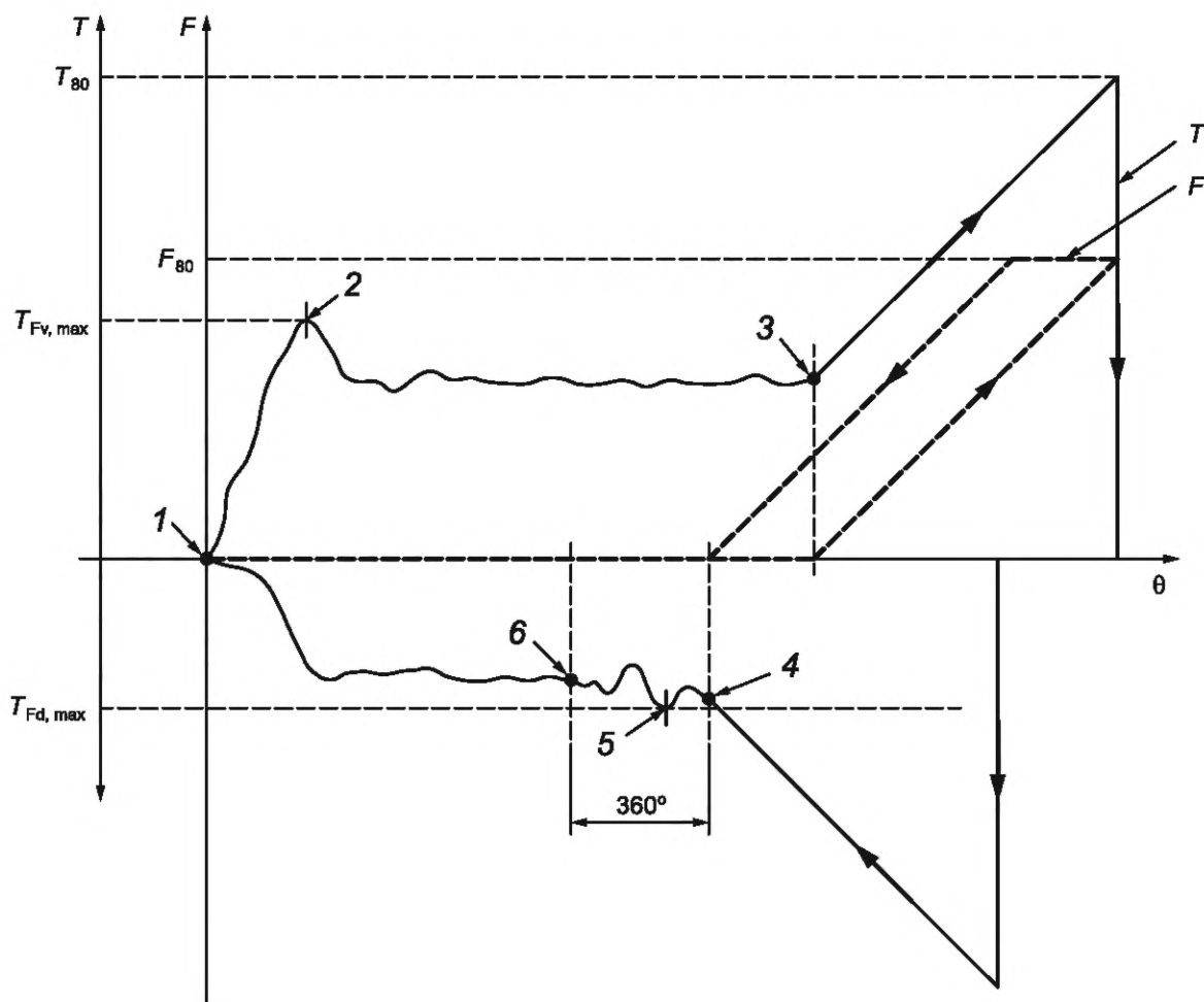
F — усилие предварительной затяжки; T — крутящий момент; \theta — угол поворота; 1 — точка, в которой впервые возникает стопорящий момент при закручивании и начинается измерение T_{Fv} ; 2 — стопорящий момент при закручивании; 3 — точка посадки, окончание измерений T_{Fv} ; 4 — отсутствие контакта с испытательной пластиной/шайбой, начало измерения T_{Fd} ; 5 — стопорящий момент при откручивании; 6 — окончание измерения T_{Fd}
