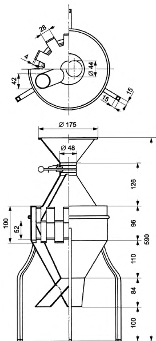
Рисунок 2 — Конический делитель
