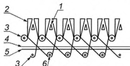
1 — разрезной прут; 2 — разрезной ворс; 3 — коренная основа; 4 — нерабочий ворс (6.8); 5 — настилочная основа; 6 — уток
