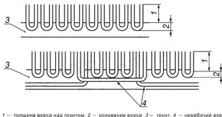
1 — толщина ворса над грунтом; 2 — основание ворса; 3 — грунт; 4 — нерабочий ворс
