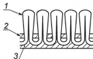
1 — петлевой ворс; 2 — грунтовая ткань; 3 — покрытие
