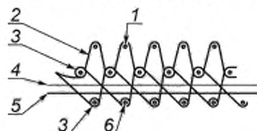
1 — петлевой прут; 2 — петлевой ворс; 3 — коренная основа; 4 — нерабочий ворс; 5 — настилочная основа; 6 — уток
