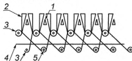
1 — разрезной прут; 2 — разрезной ворс; 3 — коренная основа; 4 — настилочная основа; 5 — уток
