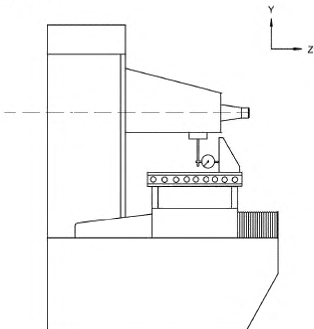
Схема измерений
