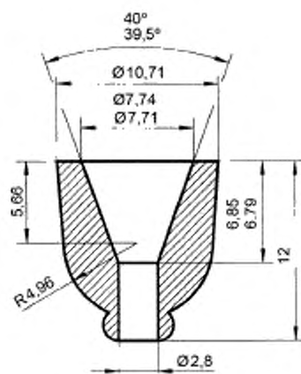
Рисунок 4 — Указатель уровня погружения термометра
