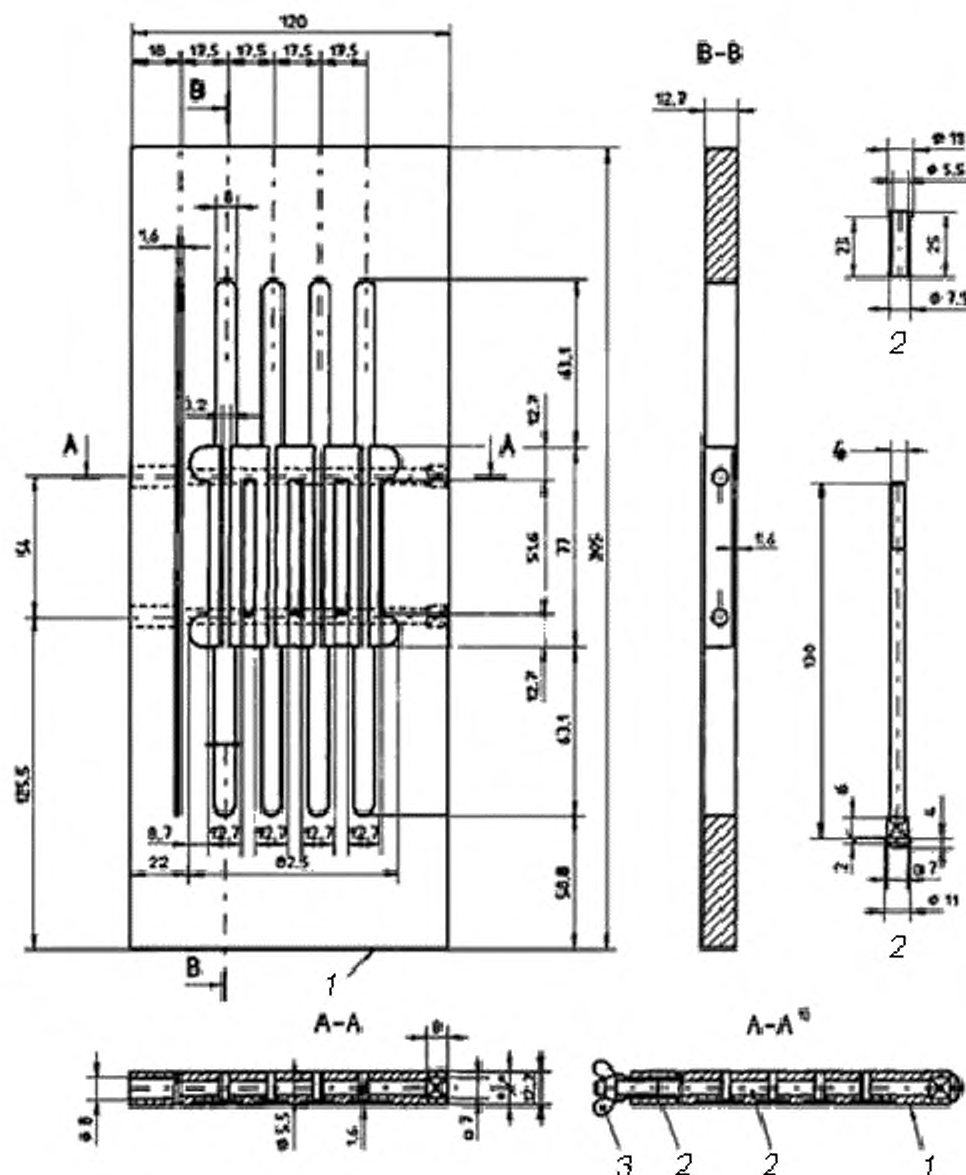
1 — пластмасса; 2 — латунь; 3 — гайка-«барашка» (крыльчатая гайка); 4 — резьба M5 (или эквивалентная)
