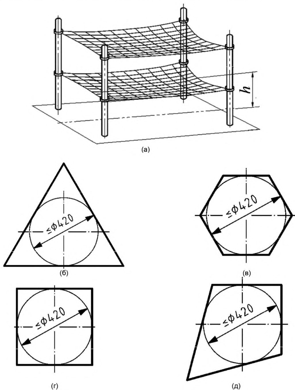
а — пространственная игровая сеть с горизонтальными плоскостями; б, в, г, д — требование к диаметру ячеек
