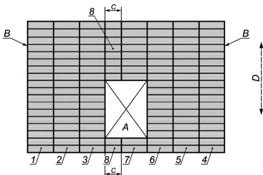
A — нарушение направления; B — стена; C — обрезанная ширина; D — направление укладки; 1—8 — полосы текстильного напольного покрытия
