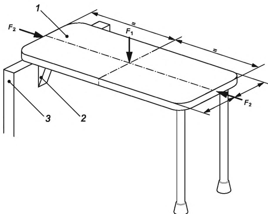
Рисунок 40 — Метод испытания держателей для переносной скамьи на прочность
