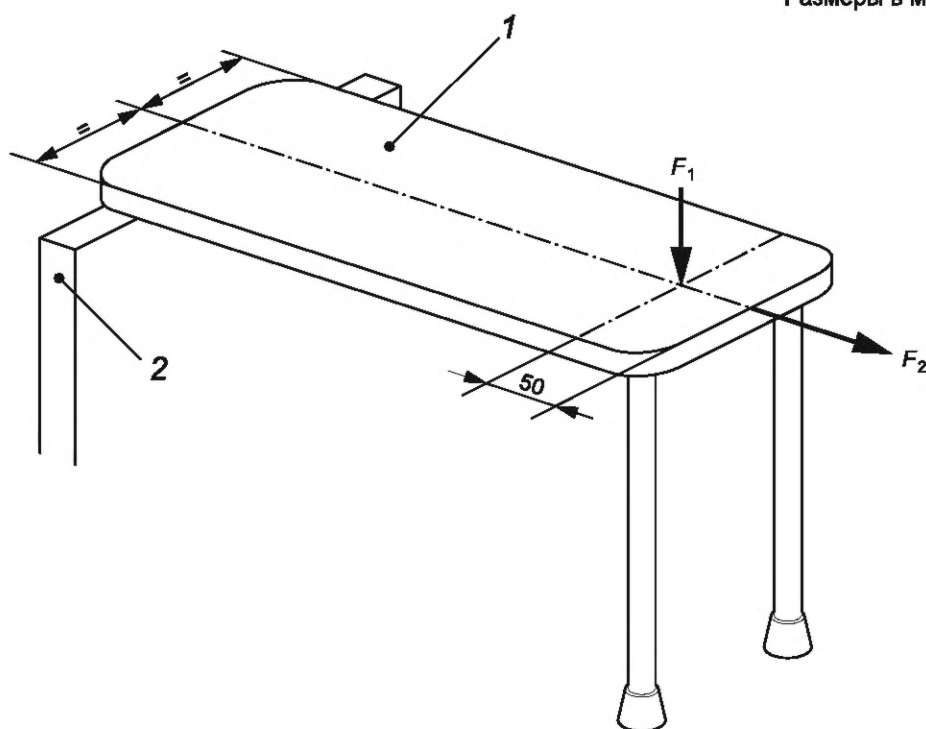
1 — переносная скамья для ванны; 2 — опорная стойка
