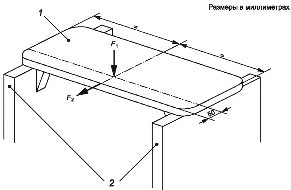
Рисунок 35 — Испытание переносной скамьи для ванны, доски для ванны и сиденья на устойчивость при движении вперед
