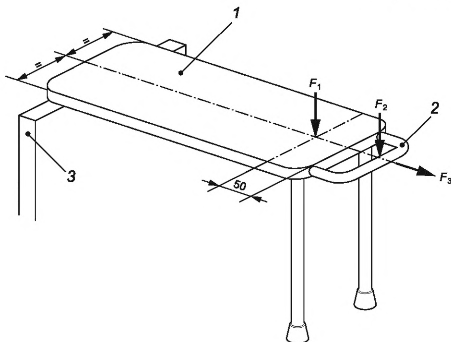
Рисунок 37 — Испытание переносной скамьи для ванны с горизонтальной ручкой на боковую устойчивость
