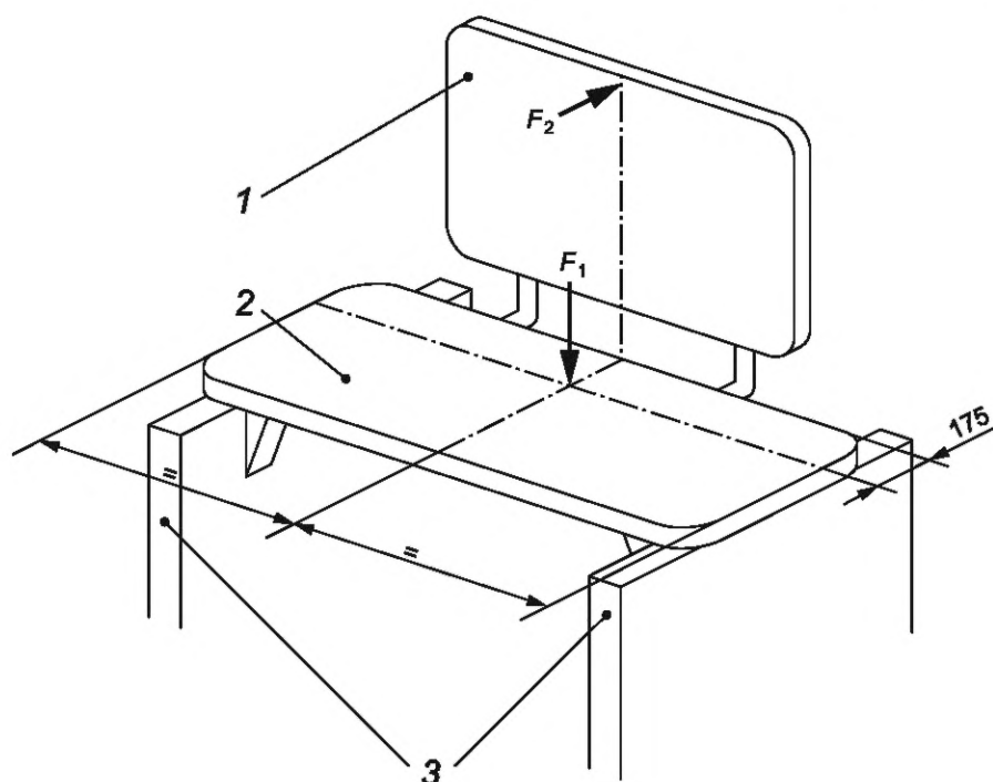
1 — переносная скамья для ванны; 2 — ручка; 3 — опорная стойка
