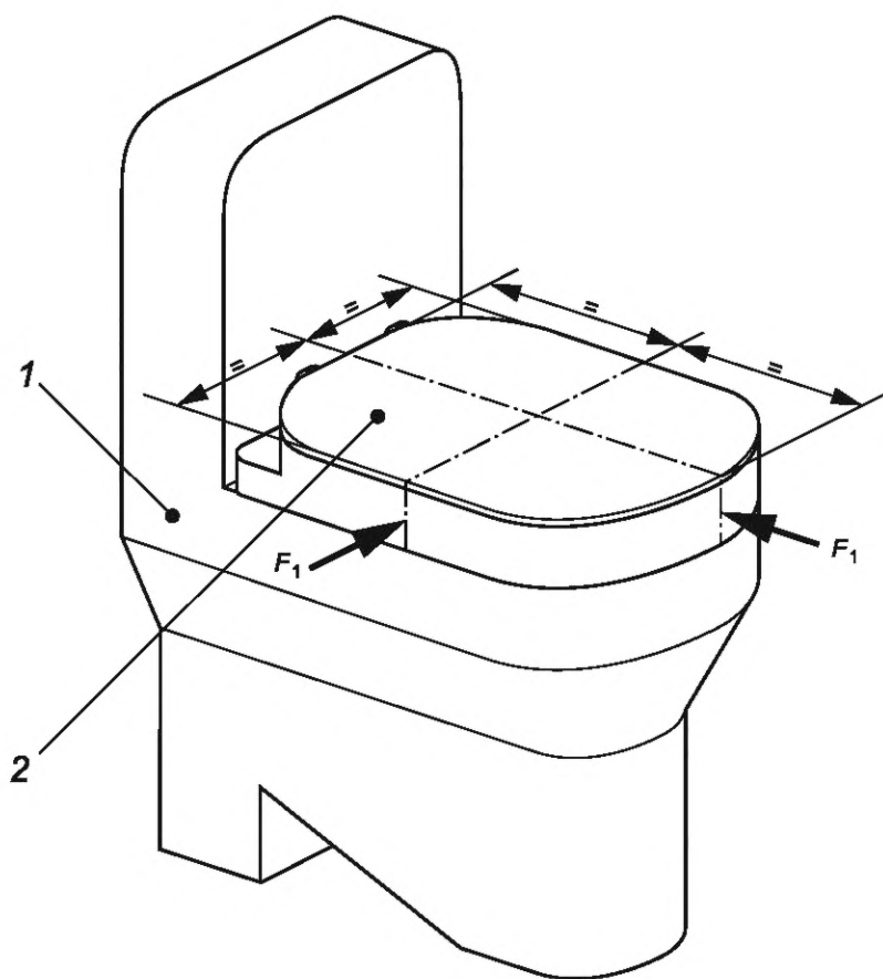
1 — стандартный туалет; 2 — сиденье унитаза
