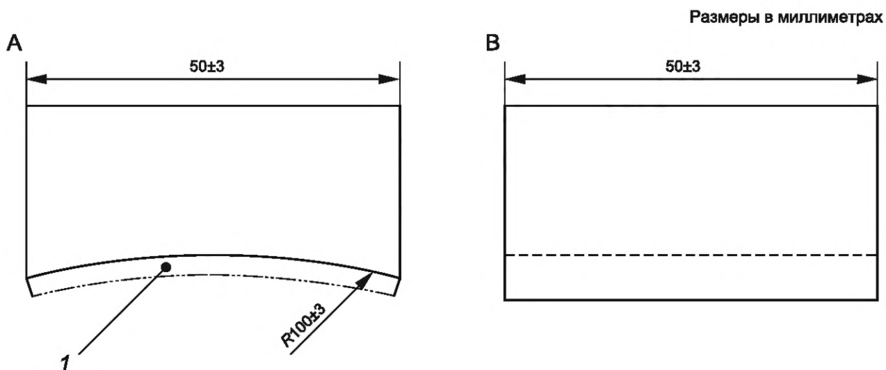
А — вид спереди; В — вид сбоку; 1 — погрузочная поверхность
