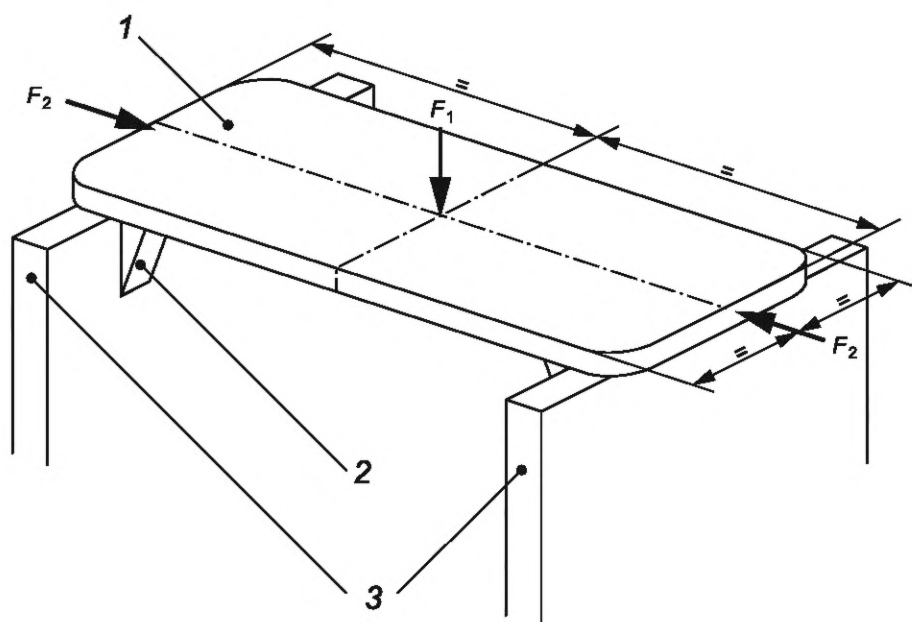
Рисунок 41 — Метод испытания держателей для бортиков/сидений для ванны на прочность
