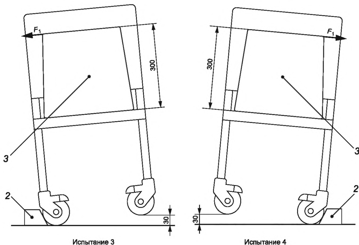
Рисунок 20 — Испытание на прочность рамы АРРН
