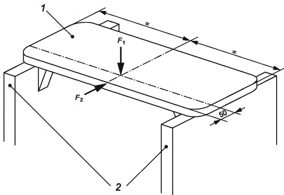
Рисунок 43 — Испытание доски для ванны на сопротивление скольжению
