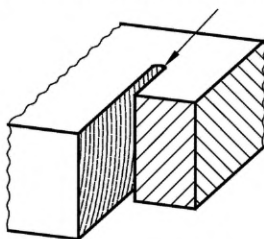
Рисунок 29 — Неполный рез в направлении резки
