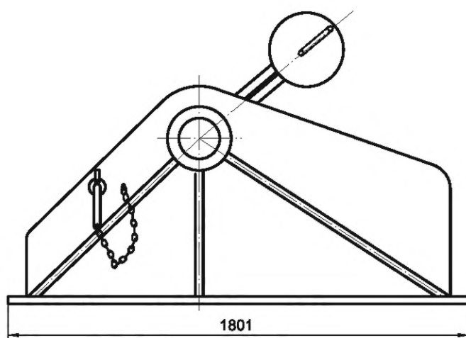
Рисунок А.3 — Цепной стопор с язычком с SWL = 350 т
