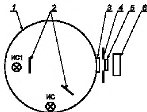
Рисунок Д.1 — Схема установки для измерения светового потока ИС, излучающих как в нижнюю, так и верхнюю полусферу
