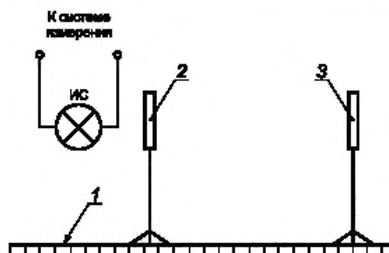
1 — фотометрическая скамья; 2 — шторка; 3 — фотометрическая головка
