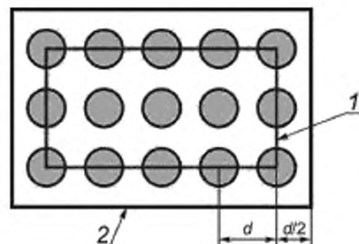
1 — периферийный многоугольник; 2 — эффективная площадь излучения
