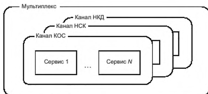
Рисунок 1 — Логическая структура мультимплекса РАВИС
