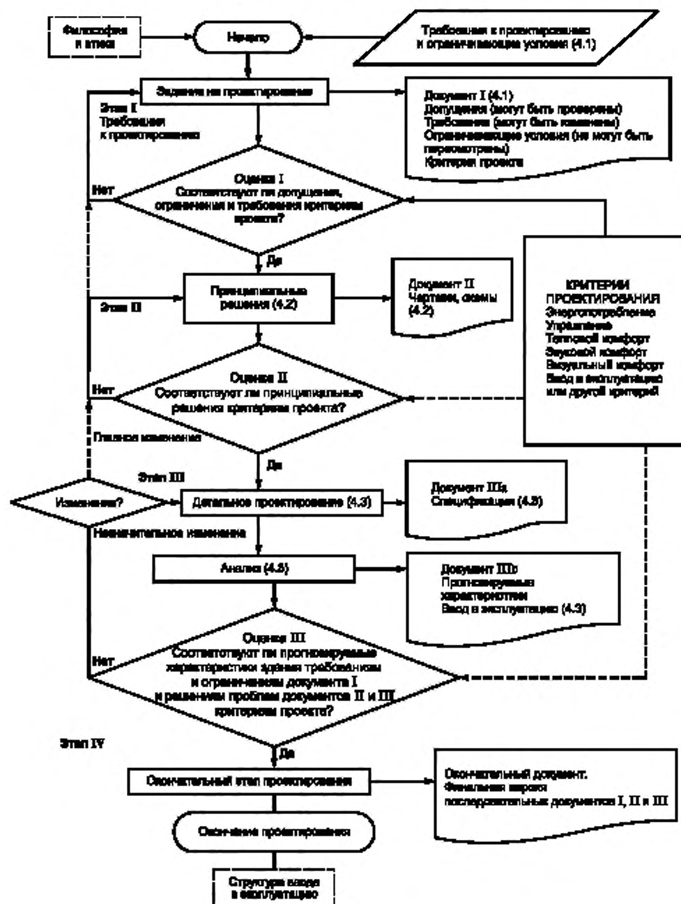
Рисунок А.1 — Диаграмма процесса проектирования
