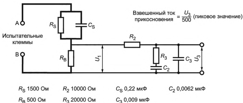
Рисунок 3 — Схема для измерения тока прикосновения \Sigma(I_A)
