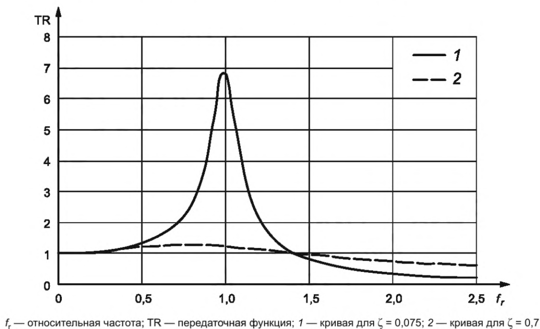
Рисунок 11 — Модуль коэффициента динамического усиления
