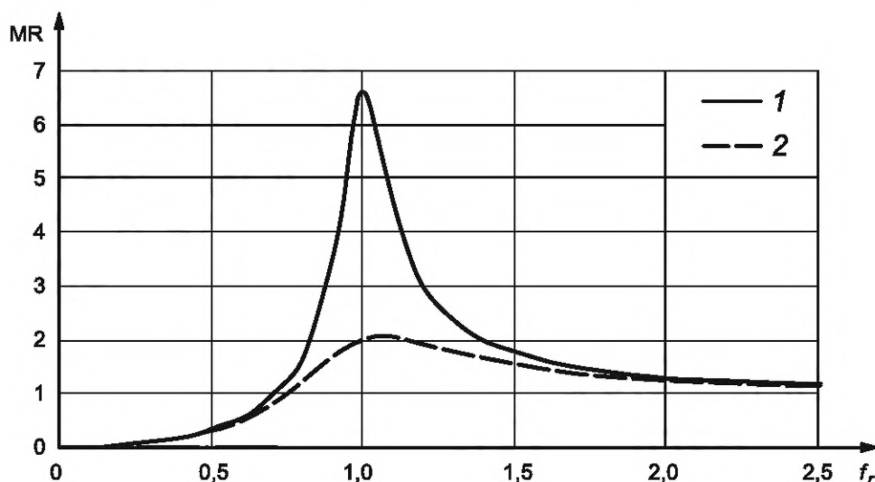
f_r — относительная частота; MR — модуль коэффициента динамического усиления для ускорения; 1 — кривая для \zeta = 0,075 ; 2 — кривая для \zeta = 0,25
