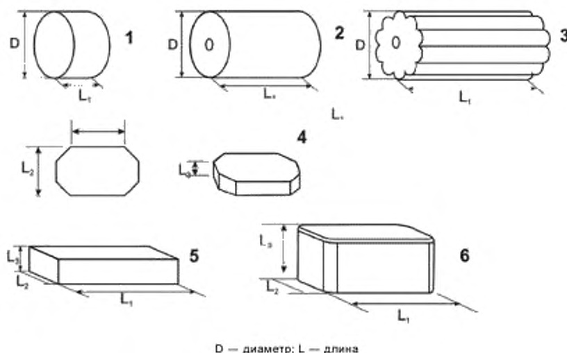
Рисунок 1 — Примеры брикетов различной формы
