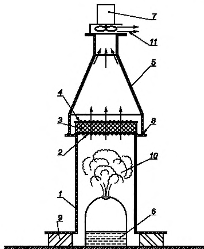
1 — воздухопроницаемая основа; 2 — нижняя опорная сетка; 3 — образец для испытаний; 4 — верхняя прижимная сетка; 5 — воздухопроницаемый короб; 6 — электропарувлажнитель; 7 — воздушный насос; 8 — резиновые уплотнители; 9 — подставки под основание; 10 — паровоздушная смесь; 11 — отработанная паровоздушная смесь
