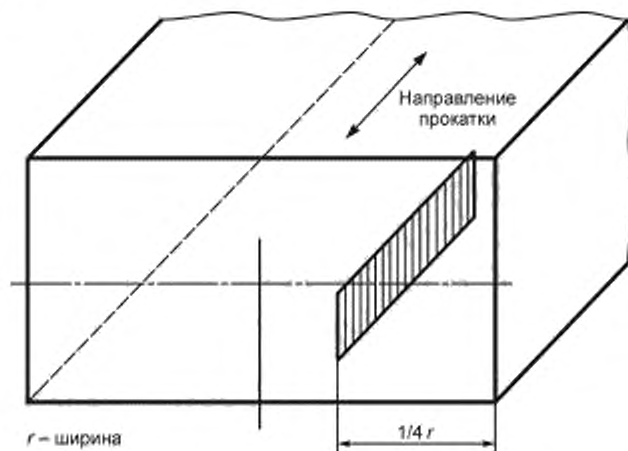
Рисунок 6 — Образец от листа толщиной свыше 50 мм
