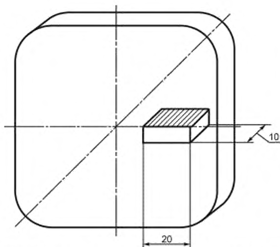
Рисунок 1 — Образец от прутка или заготовки с диаметром или длиной стороны свыше 40 мм
