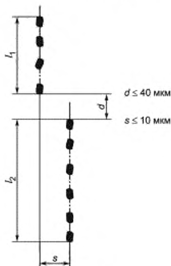
Рисунок 9 — Включения типа В
