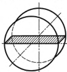
Рисунок 3 — Образец от прутка диаметром не более 25 мм
