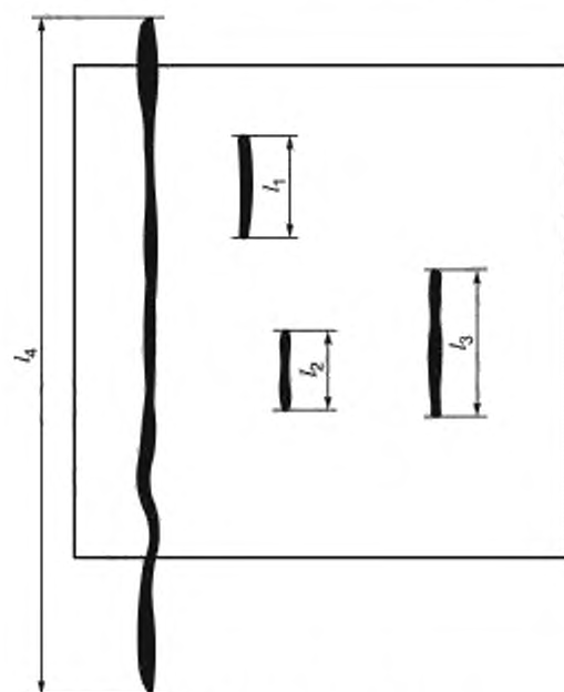
Оценка поля основана на полной длине L L = 0,71 + l_1 + l_2 + l_3 с отдельным указанием сверхразмерной длины l_4 a — Для включений или строчек сверхразмерных только по длине
