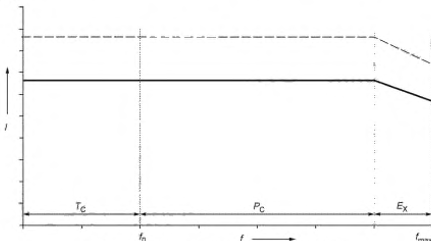
Рисунок 2 — Допустимый выходной ток преобразователя
