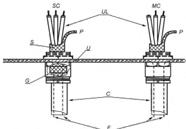
SC — питающий кабель, MC — кабель двигателя, UL — отрезок без экрана (по возможности короткий); S — экран кабеля; P — гибкий проводник (по возможности короткий); U — непроводящая плата уплотнения; G — кабельное уплотнение для электромагнитной совместимости; C — кабели (внешняя оболочка); F — непрерывная клетка Фарадея
