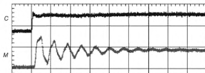
C — фазное напряжение преобразователя; M — фазное напряжение двигателя
