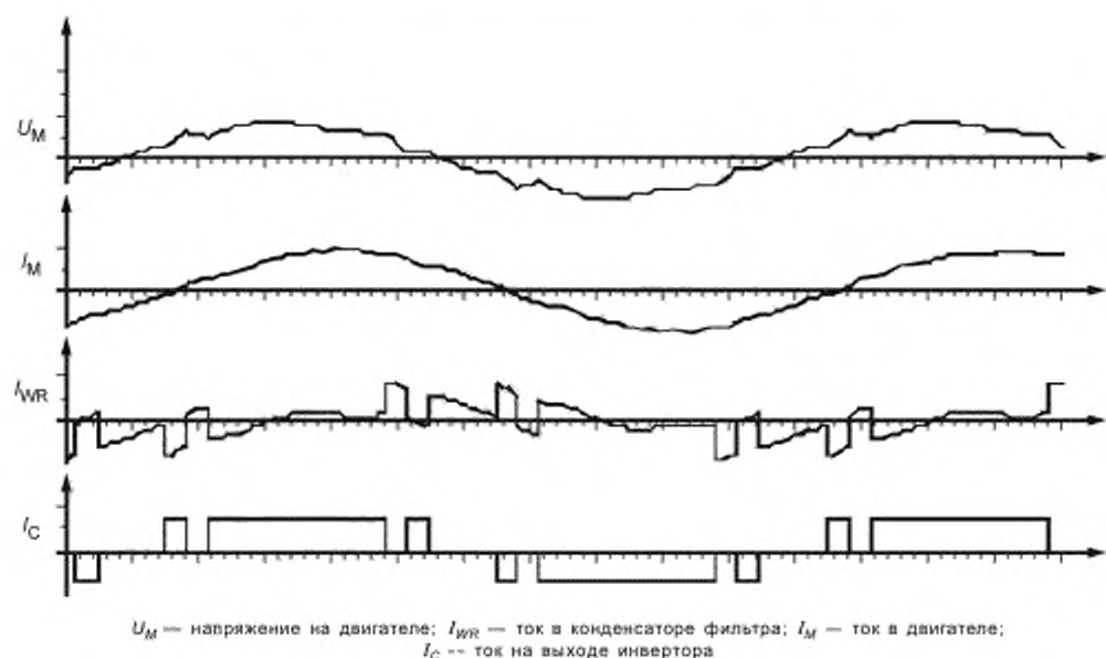
Рисунок 34 — Кривые напряжений и токов системы с ШИМ-инвертором тока
