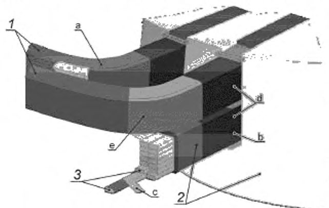
1 — межфазная изоляция; 2 — изоляция фазы относительно земли; 3 — межвитковая изоляция, а — фазная изоляция/изоляция конца обмотки; б — изоляция на землю; в — витковая изоляция, д — слой, сдерживающий пазовое перенапряжение, е — слой, контролирующий перенапряжение на конце обмотки (выравнивание перенапряжений)
