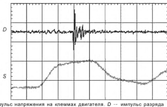
S — импульс напряжения на клеммах двигателя. D — импульс разряда Рисунок 13 — Импульс разряда на клеммах двигателя (100 нс/деление)
