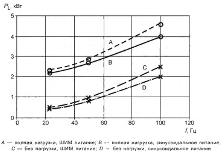
Рисунок 4 — Зависимость измеренных потерь P_L от частоты f , нагрузки и типа питания
