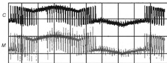
C — фазное напряжение преобразователя; M — фазное напряжение двигателя
