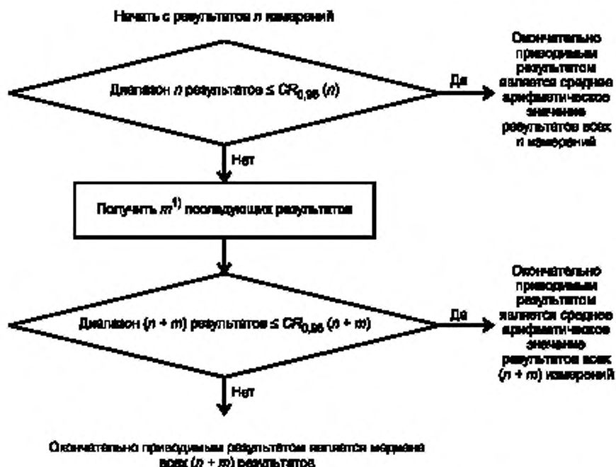
Рисунок 6 — Метод проверки приемлемости результатов измерений, полученных в условиях повторяемости, при n \geq 5 и условии, что получение результатов измерений не является дорогостоящим, или при n \geq 4 и при условии, что получение результатов измерений является дорогостоящим (вариант С)
