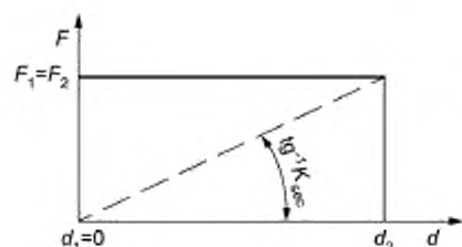
Рисунок D.2 — Жесткопластические устройства
