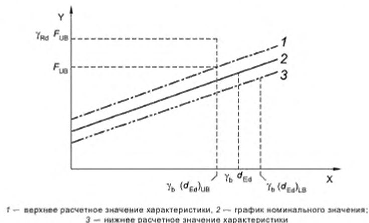
Рисунок Н.2 — Схематическая диаграмма, показывающая определение F_{UB} для скользящих опор
