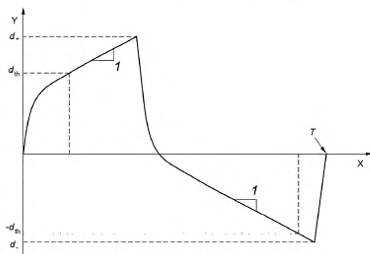
Рисунок Е.5 — График нагружения для испытаний при низкой скорости
