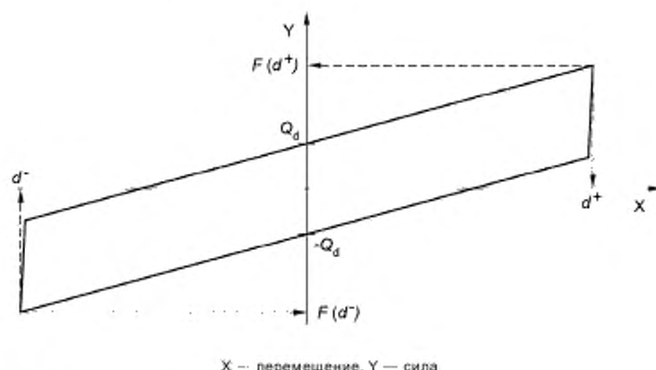
Рисунок G.1 — Схематическая петля гистерезиса сила — перемещение для эластомерных опор со свинцовым сердечником
