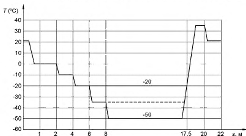
Рисунок 6 — Пример температурной программы длительного испытания трения скольжения для T_{\min} = -50^{\circ}\text{C} и T_{\min} = -20^{\circ}\text{C}
