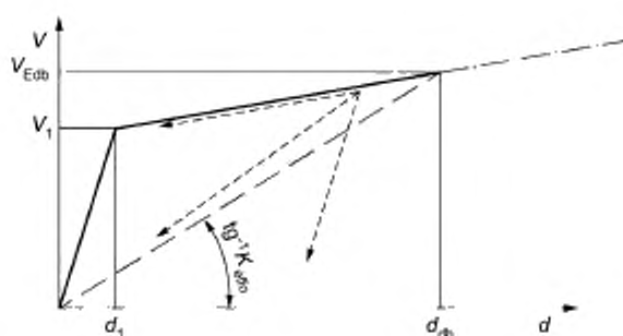
Рисунок 2 — Эффективная жесткость нелинейного устройства
