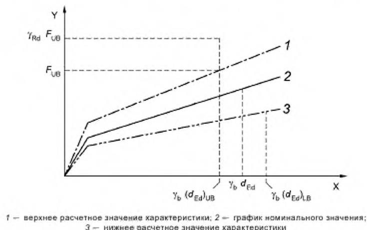
Рисунок Н.1 — Схематическая диаграмма, показывающая определение F_{UB} для эластомерных сейсмоизоляторов
