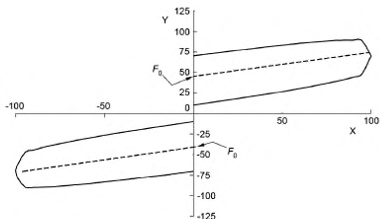
Рисунок Е.2 — Огибающая кривой зависимости силы от перемещения жидкостно-пружинного демпфера (синусоидальная нагрузка)
