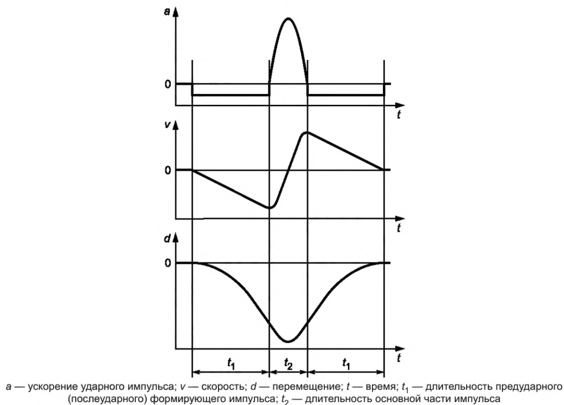
Рисунок А.1 — Сигналы ускорения, скорости и перемещения для импульса полусинусоидальной формы
