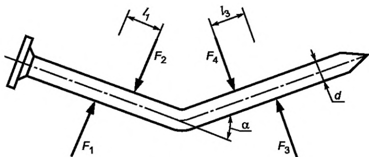
Рисунок 2 — Деформация гвоздя
