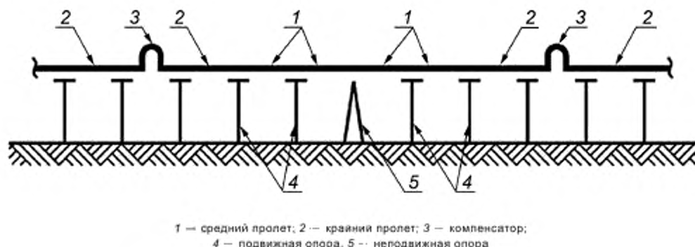
Рисунок 1 — Конструкции опор надземного перехода газопровода
