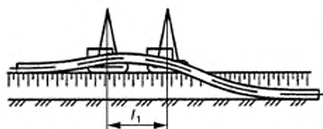
l_1 — расстояние между кранами-трубоукладчиками
