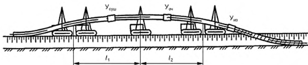
Y_{\text{суш}} — установка сушильная; Y_{\text{оч}} — установка очистки; Y_{\text{из}} — установка изоляционная; l_1, l_2 — расстояния между кранами-трубоукладчиками
