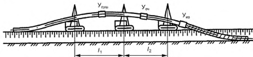
Рисунок Б.14 — Совмещенный способ изоляции и укладки газопровода номинальным диаметром свыше DN 500 до DN 800 включительно
