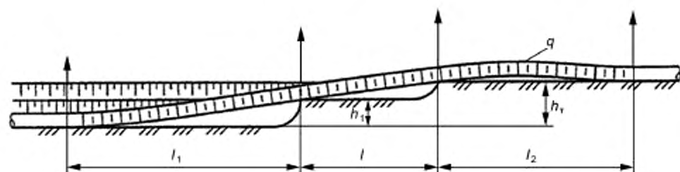
Рисунок Б.17 — Расчетно-технологическая схема укладки газопровода за один проход методом «подкоп»
