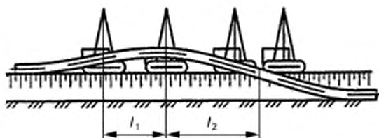
l_1, l_2 — расстояния между кранами-трубоукладчиками
