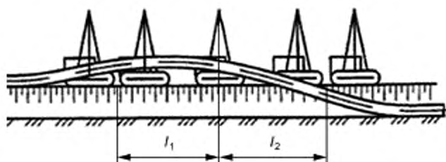
l_1, l_2 — расстояния между кранами-трубоукладчиками
