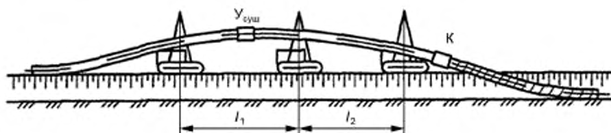
Y_{суш} — установка сушильная; К — комбайн для очистки и изоляции газопровода, l_1, l_2 — расстояния между кранами-трубоукладчиками
