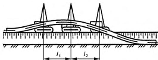
l_1, l_2 — расстояния между кранами-трубоукладчиками
