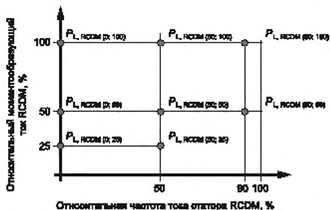
Рисунок 6 — Опорные рабочие точки (относительная частота тока статора и ток статора) для определения относительных потерь эталонного комплектного преобразователя (RCDM)
