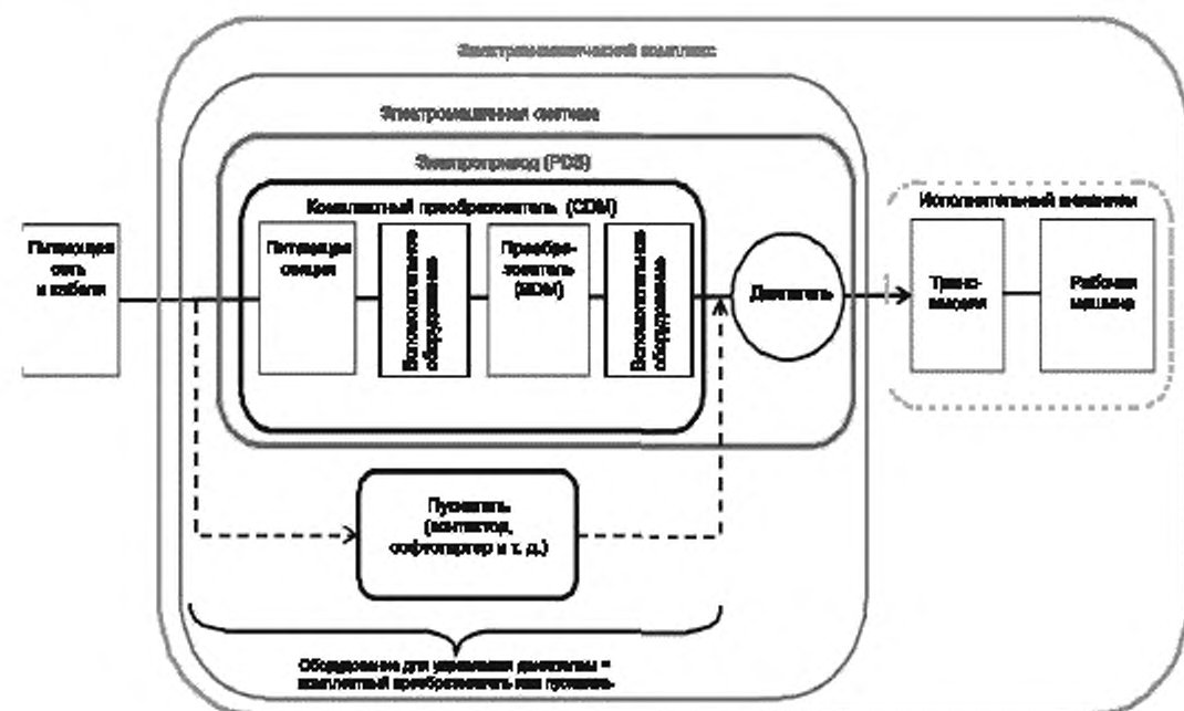
Рисунок 2 — Электромеханический комплекс
