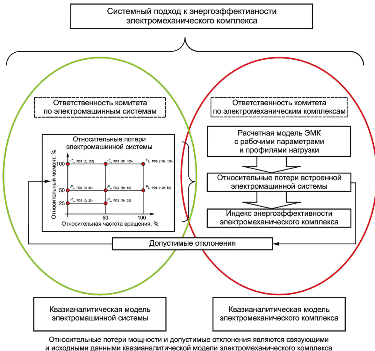
Рисунок 6 — Ответственность и процедуры при определении индекса энергоэффективности электромеханического комплекса
