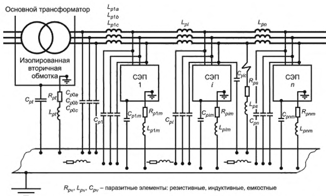
Рисунок D.3 — Безопасность и применение фильтров
