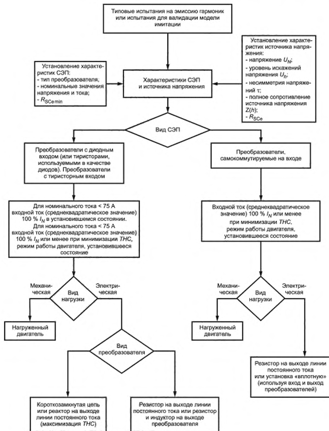
Рисунок В.5 — Условия нагрузки при измерении гармонических составляющих, создаваемых СЭП
