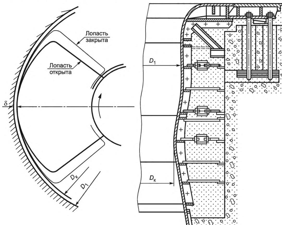
Рисунок Б.3.1 — Схема измерения зазора «камера — лопасть» для гидротурбин поворотно-лопастного типа
