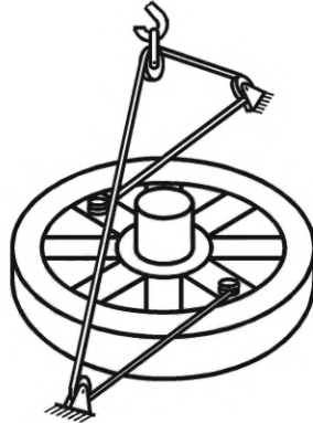
Рисунок Е.2.3 — Симметричный способ поворота ротора ГА
