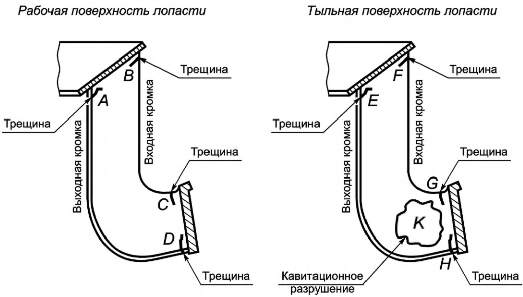
Кавитационные повреждения
