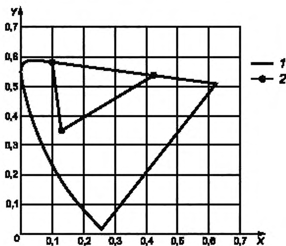
x, y — координаты цветности; 1 — линия спектральных цветностей; 2 — OLED (типовая)
