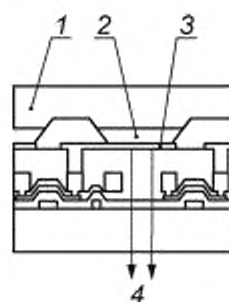
OLED с излучением снизу
