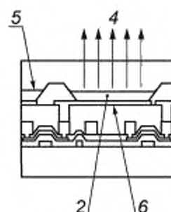
OLED с излучением сверху
