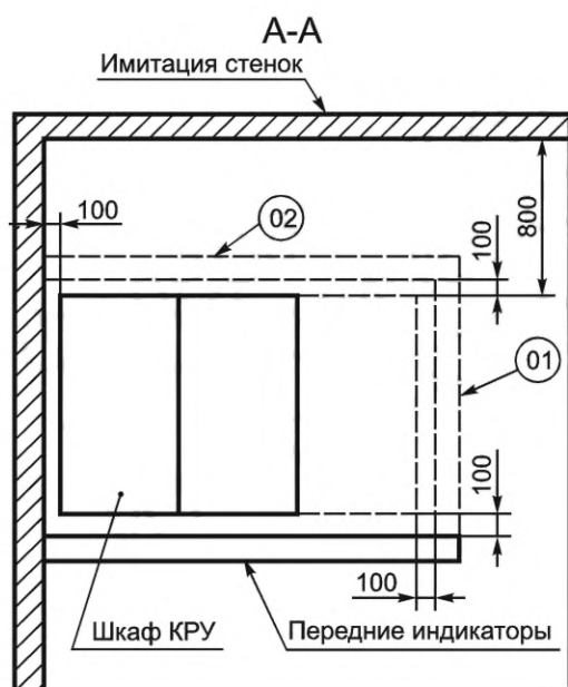
Рисунок А.6 — Имитация помещения и положение индикаторов для типа доступа В, высота шкафов КРУ менее 2,0 м
