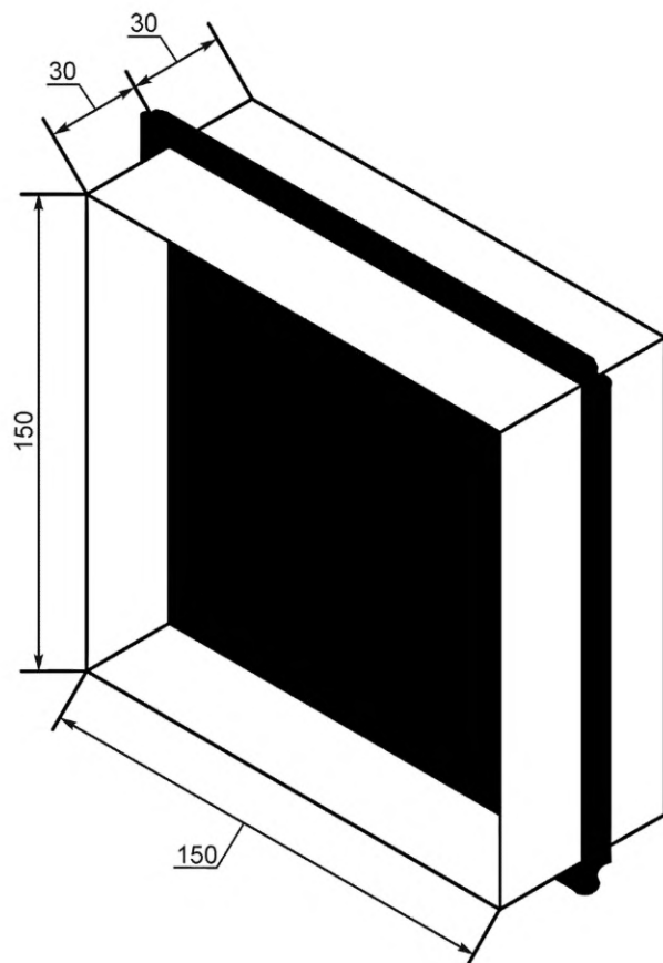
Рисунок А.1 — Монтажная рамка для вертикального индикатора (размеры в миллиметрах)
