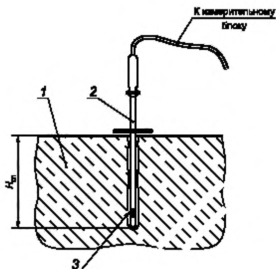
1 — контролируемый материал; 2 — зондовый датчик; 3 — чувствительный элемент; H_{гп} — глубина скважины
