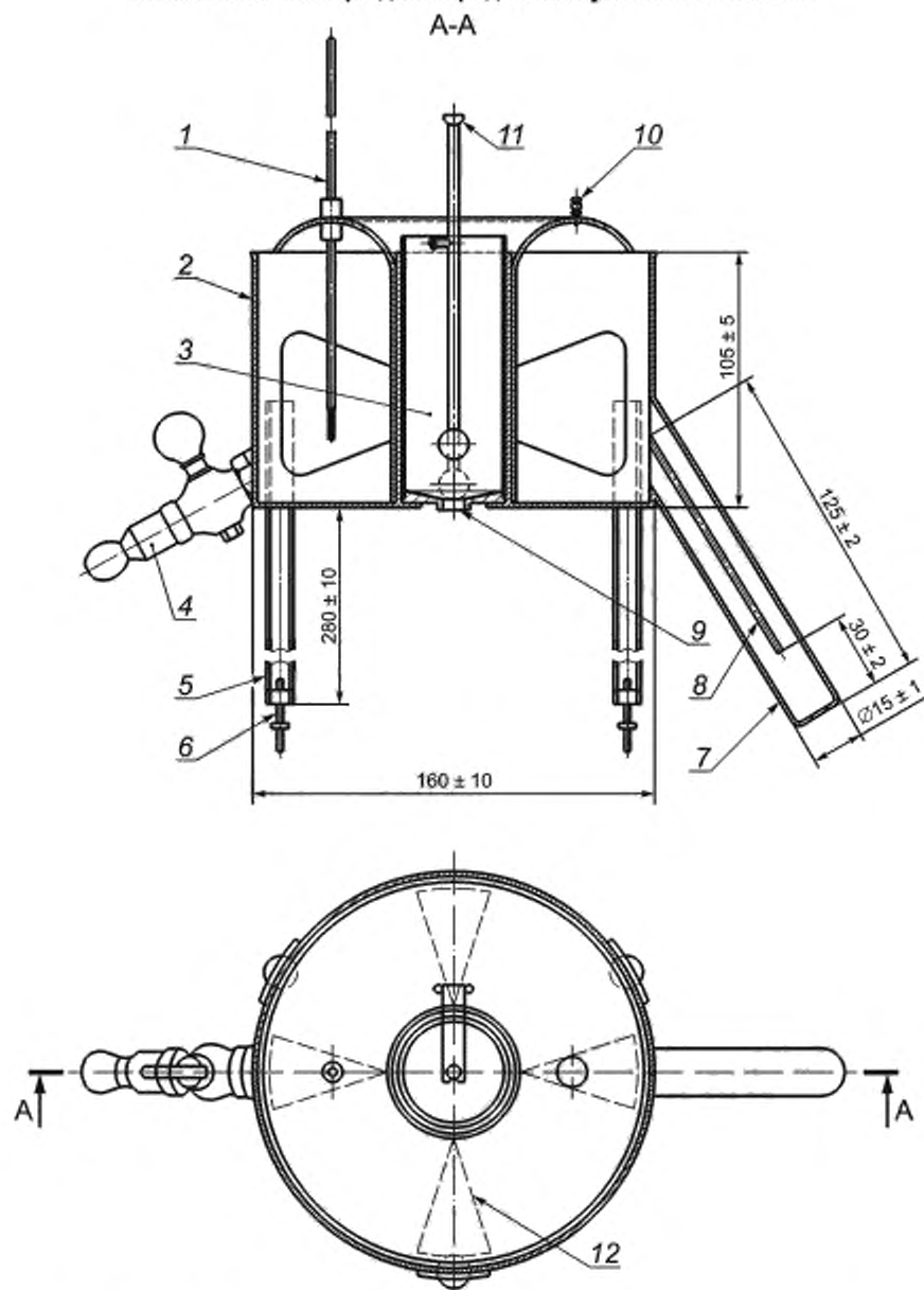
Схема вискозиметра для определения условной вязкости
