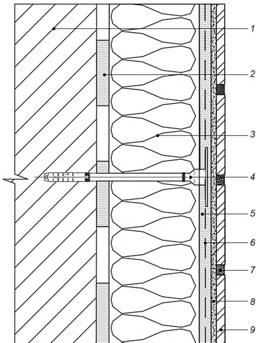
1 — основание (стена); 2 — клеевой слой; 3 — теплоизоляционный слой; 4 — анкер с тарельчатым дюбелем; 5 — армированный базовый слой, усиленный фасадной стеклосеткой; 6 — фасадная стеклосетка; 7 — затирочный шов; 8 — клеевой плиточный слой; 9 — элементы (плитка) декоративно-защитного слоя
