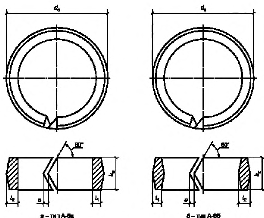
Рисунок А.6 — Схема кольцевых шлонок типа А-6
