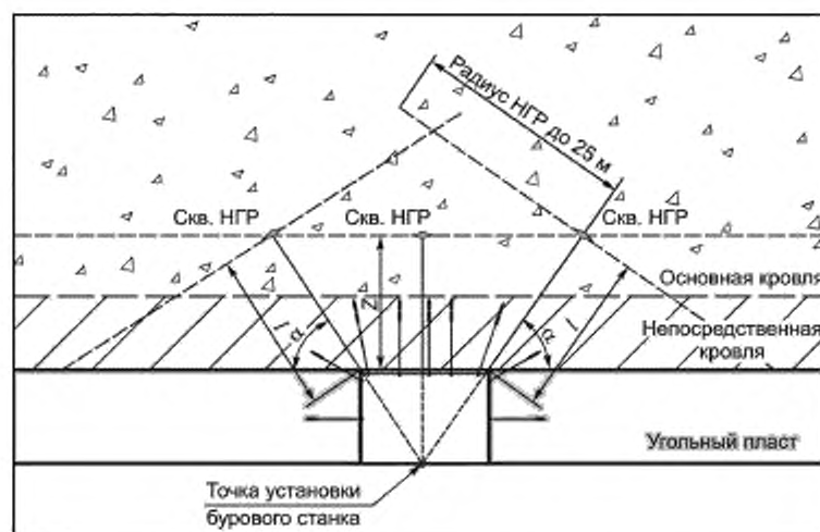
Рисунок 1 — Общая схема расположения скважин НГР
