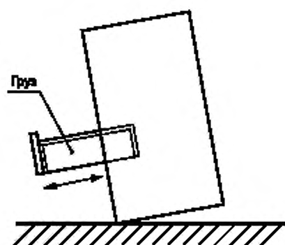
Рисунок 2 — Испытания на сопротивление самопроизвольному выдвижению выдвижного ящика (выдвижной полки) из корпуса тумбы
