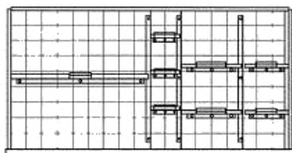
Рисунок Б.3 — Примеры видов перегородок, размещаемых в выдвижных ящиках (на выдвижных полках)
