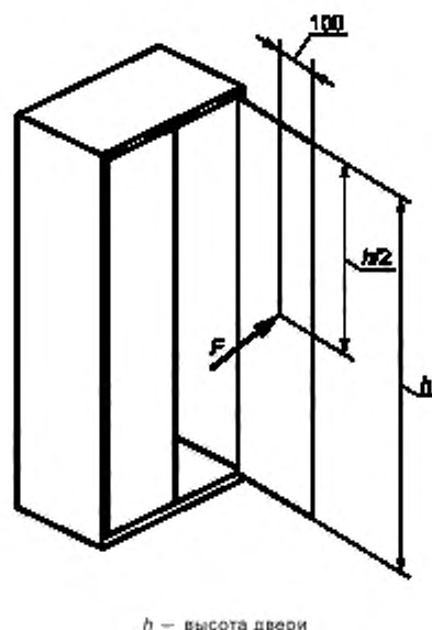
Рисунок 5 — Испытания распашных дверей горизонтальной статической нагрузкой
