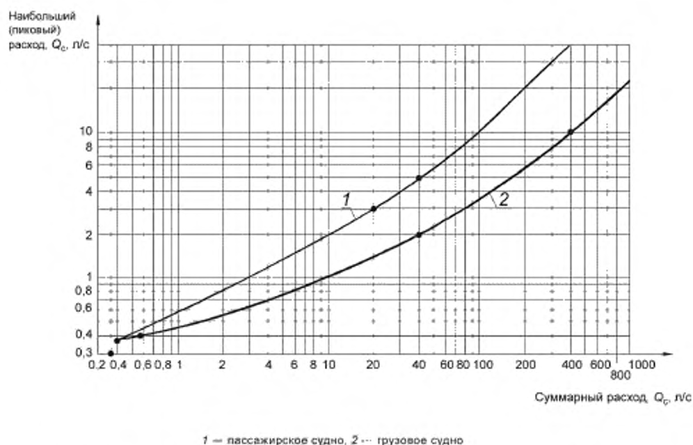
Рисунок Г.1 — График для определения наибольшего (пикового) расхода питьевой воды в зависимости от суммарного расхода воды
