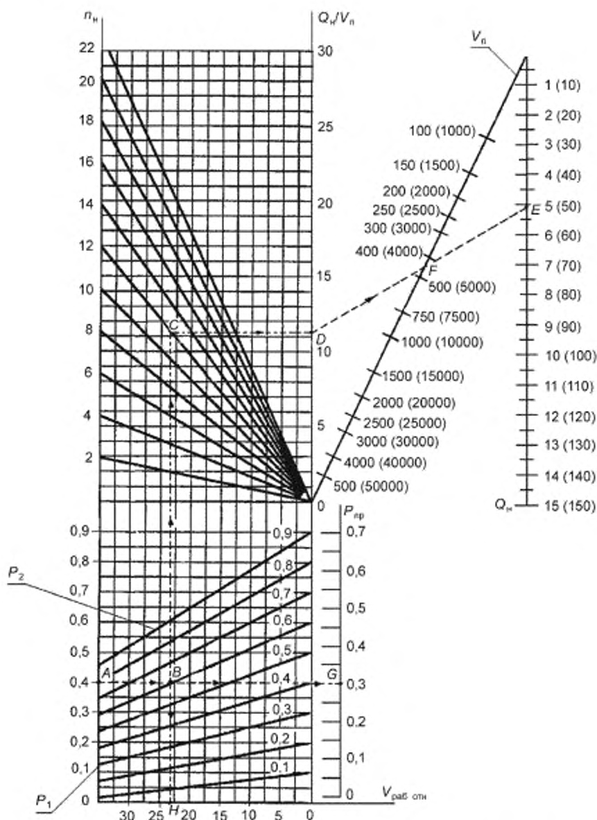
Рисунок E.3 — Номограмма для определения объема пневмоцистерны
