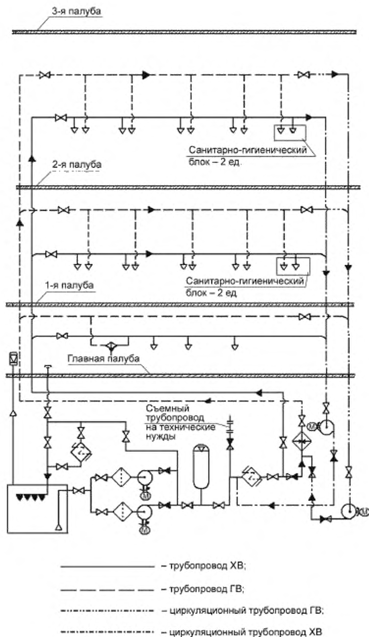
Рисунок 1 — Принципиальная схема системы питьевой воды
