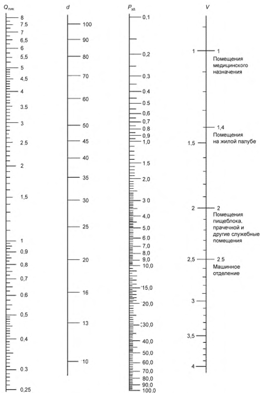
Рисунок Г.2 — Номограмма для определения номинальных диаметров трубопроводов и удельных потерь давления в зависимости от наибольшего (пикового) расхода и расчетной скорости потока воды
