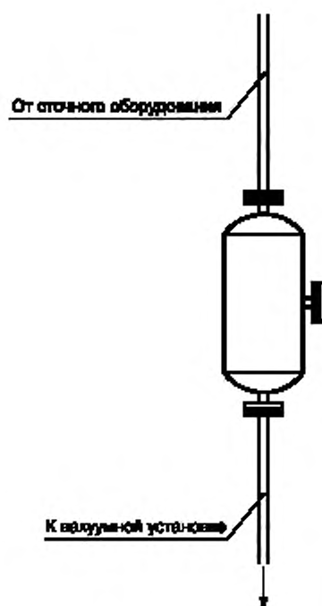
Рисунок 3 — Вакуумная емкость
