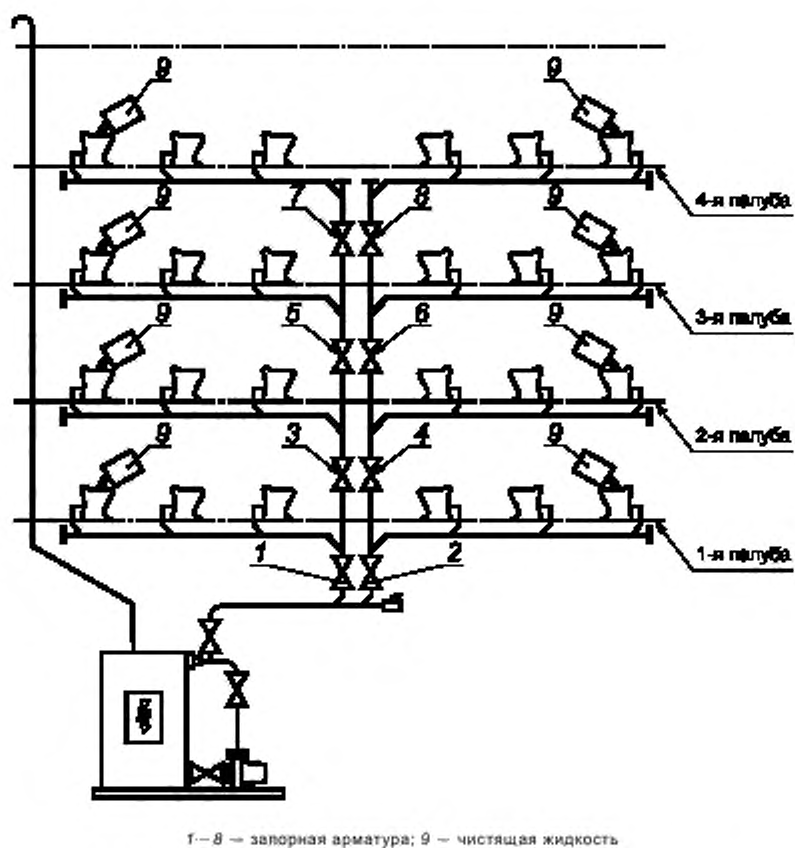
Рисунок Б.3 — Вакуумная стонная система с запорной арматурой между палубами с применением чистящей жидкости
