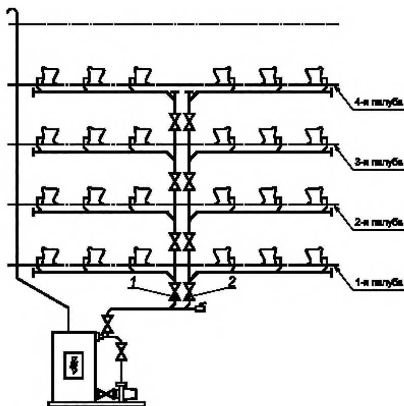
1, 2 — запорная арматура
