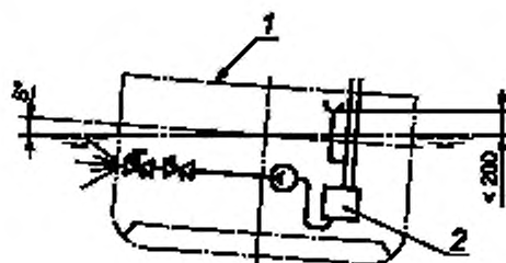
1 — палуба надводного борта; 2 — накопитель сточных вод
