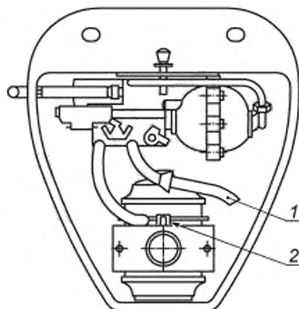
1 — трубопровод управления; 2 — запирающая крышка
