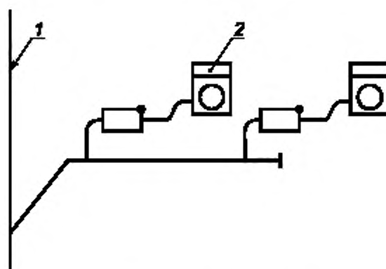
1 — коллекторный трубопровод; 2 — стиральная машина
