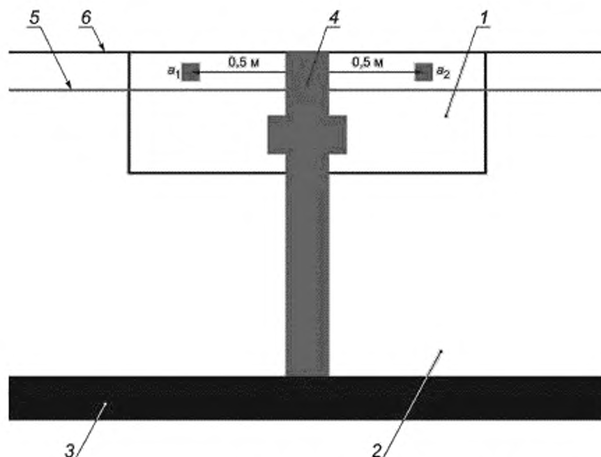
1 — контактная панель на торцевой стенке ванны; 2 — вода; 3 — дно ванны; 4 — разметка на торцевой стенке ванны; 5 — поверхность воды; 6 — верхний край контактной панели; а, и а 2 — метки пар точек на торцевой стенке ванны
