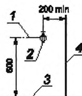
1 — горизонтальная ось водоразборного крана; 2 — водоразборный кран; 3 — палуба; 4 — боковая стенка
