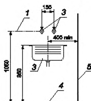
Рисунок 1 — Расположение раковины и смесителя
