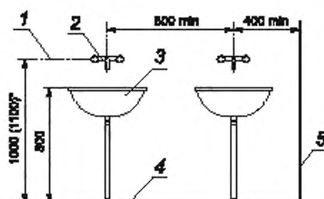
Рисунок 1 — Расположение раковины и смесителя
