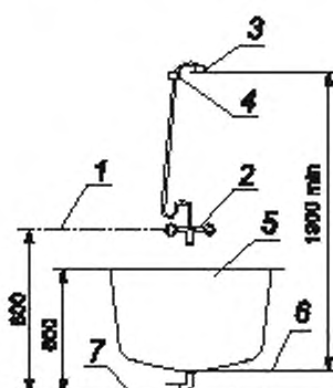
Рисунок 2 — Расположение мойки и индивидуальных водоразборных кранов или смесителя
