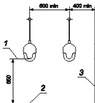
1 — уровень борта писсуара; 2 — палуба; 3 — боковая стенка
