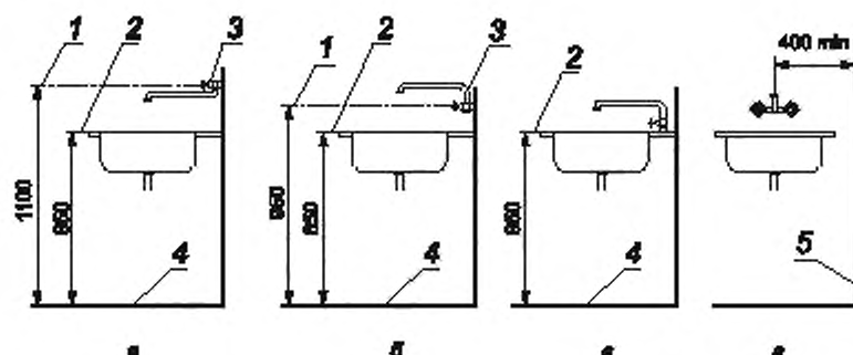
Рисунок 1 — Расположение раковины и смесителя
