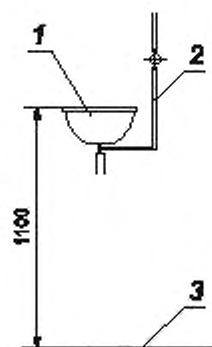
1 — питьевой фонтанчик; 2 — трубопровод питьевой воды; 3 — палуба
