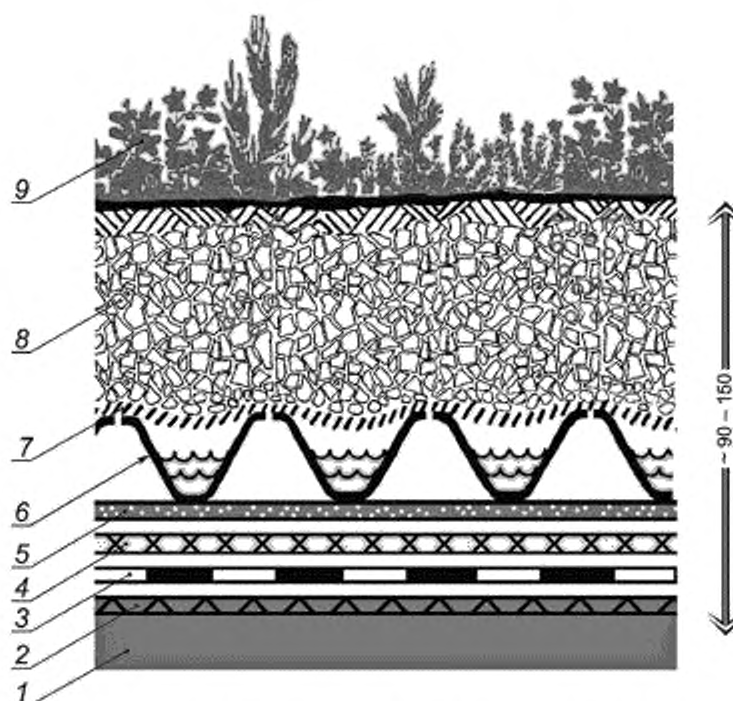
1 — несущая конструкция крыши; 2 — водоизоляционный слой; 3 — защитный слой; 4 — корнесащитный слой; 5 — влагонакопительный слой; 6 — дренажный слой; 7 — фильтрующий слой; 8 — субстрат; 9 — растительный слой
