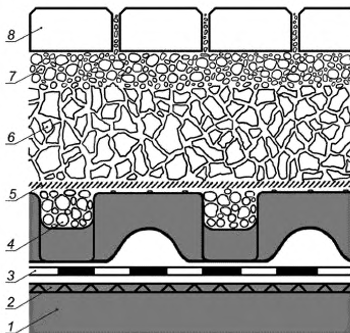
1 — несущая конструкция крыши; 2 — водоизоляционный слой; 3 — защитный слой; 4 — дренажный слой; 5 — фильтрующий слой; 6 — гранитный щебень; 7 — гранитный отсеб; 8 — плитка, брусчатка
