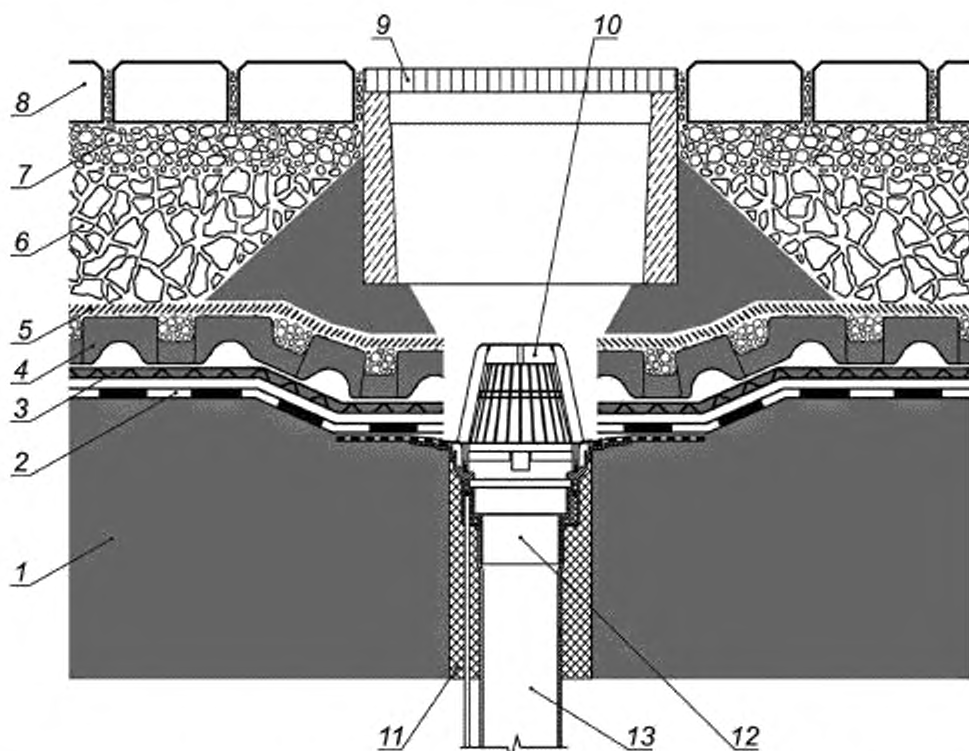
1 — несущая конструкция крыши; 2 — водоизоляционный слой; 3 — защитный слой; 4 — дренажный слой; 5 — фильтрующий слой; 6 — гранитный щебень; 7 — гранитный отсев; 8 — плитка, брусчатка; 9 — бетонный дождеприемный колодец с решеткой; 10 — листвоуловитель воронки; 11 — монтажная лена; 12 — корпус водоприемной воронки; 13 — водосточная труба
