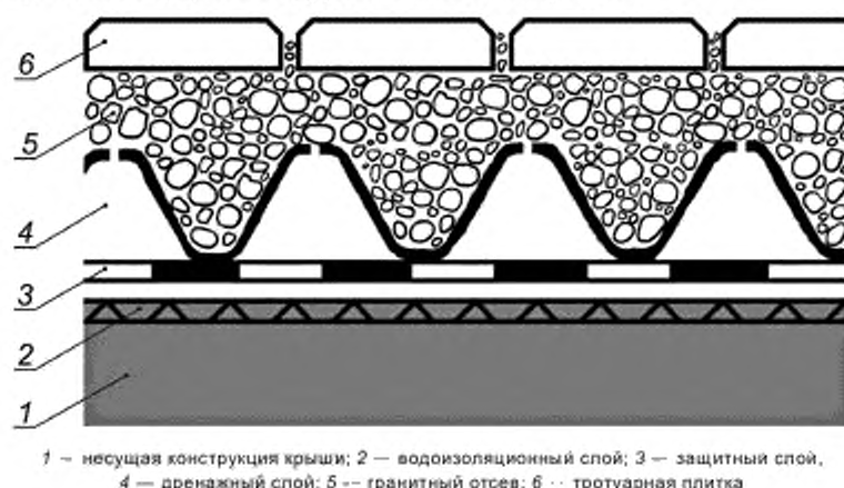
Рисунок 8 — Покрытие под пешеходную нагрузку
