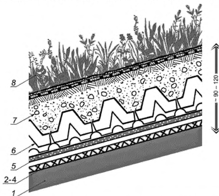
1 — несущая конструкция крыши; 2—4 — водонепроницаемый, корнезащитный слой «два в одном»; 5 — теплоизоляционный слой; 6 — дренажный слой; 7 — субстрат; 8 — растительный слой
