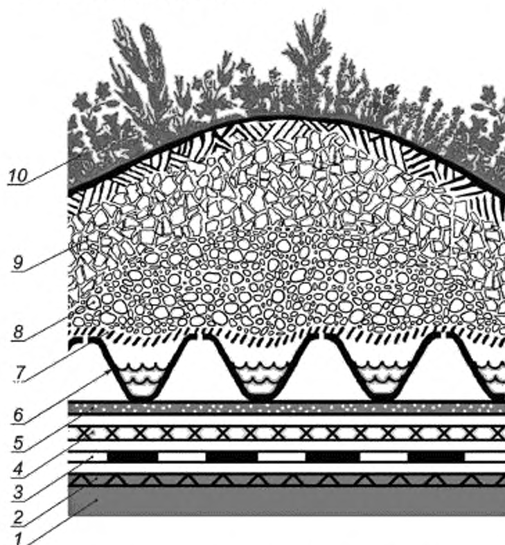
1 — несущая конструкция крыши; 2 — водоизоляционный слой; 3 — защитный слой; 4 — корнезащитный слой; 5 — влагонакопительный слой; 6 — дренажный слой; 7 — фильтрующий слой; 8 — керамзитовый гравий; 9 — субстрат; 10 — растительный слой
