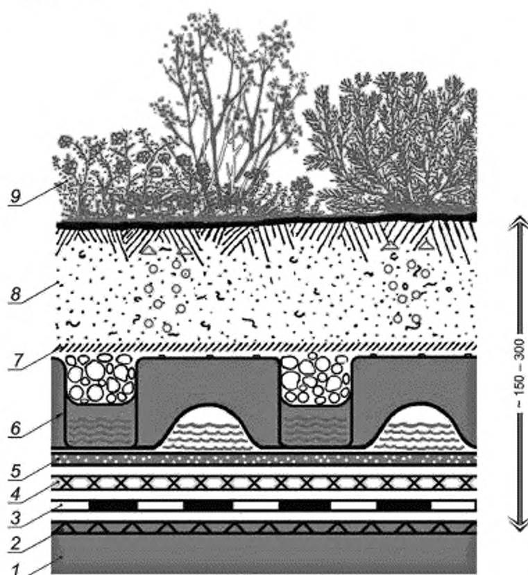
1 — несущая конструкция крыши; 2 — водоизоляционный слой; 3 — защитный слой; 4 — корневозащитный слой, 5 — влагонакопительный слой; 6 — дренажный слой; 7 — фильтрующий слой; 8 — субстрат; 9 — растительный слой
