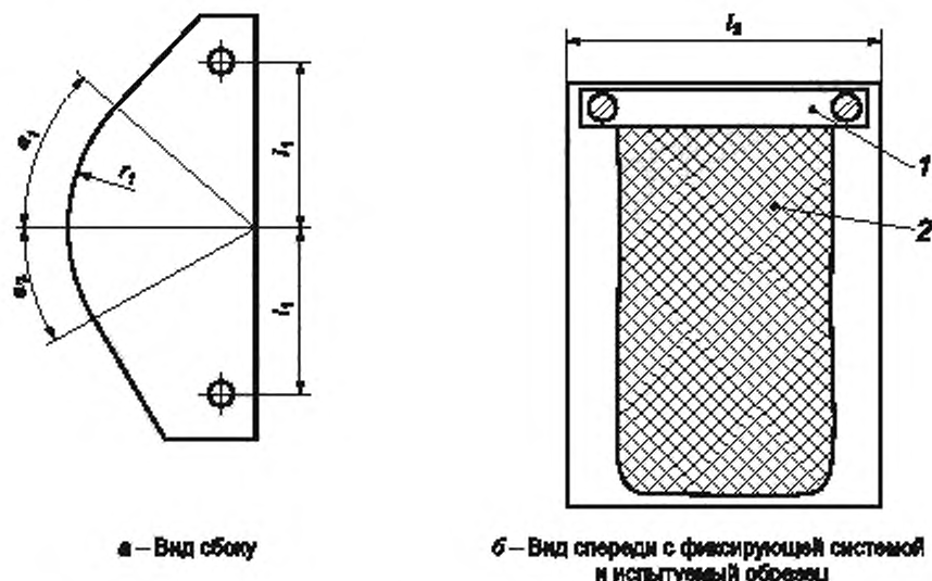
Рисунок Б.2 — Макет, несущий испытуемый образец
