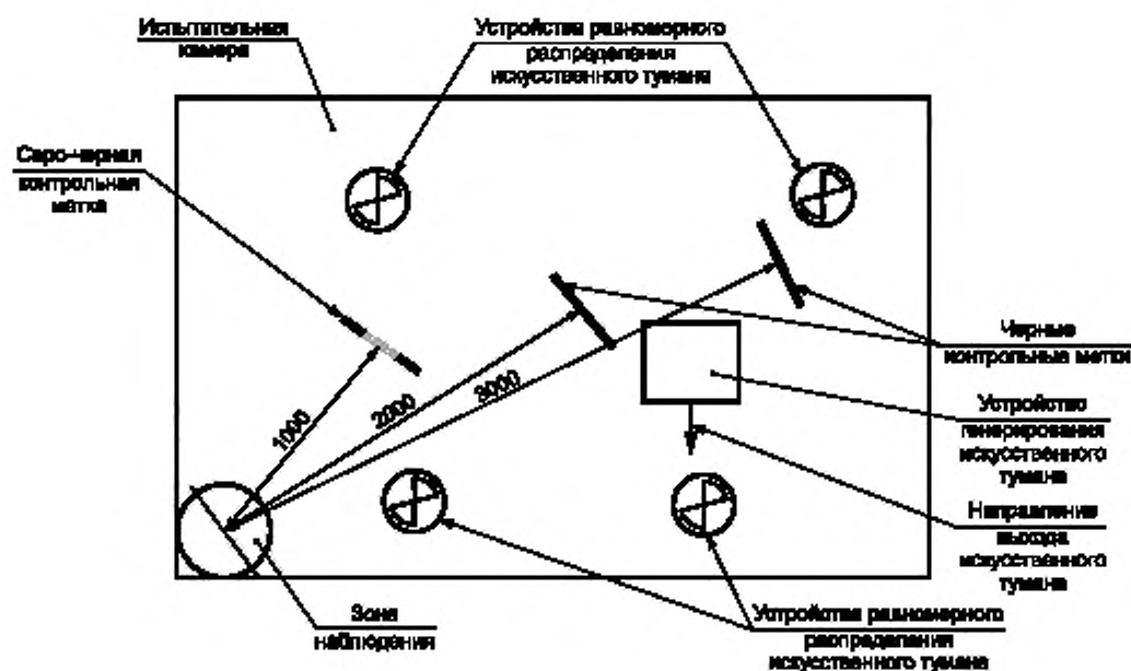
Рисунок А.1 — Рекомендуемое размещение оборудования
