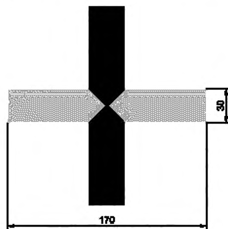
Рисунок А.2 — Рекомендуемый вид серо-черной контрольной метки
