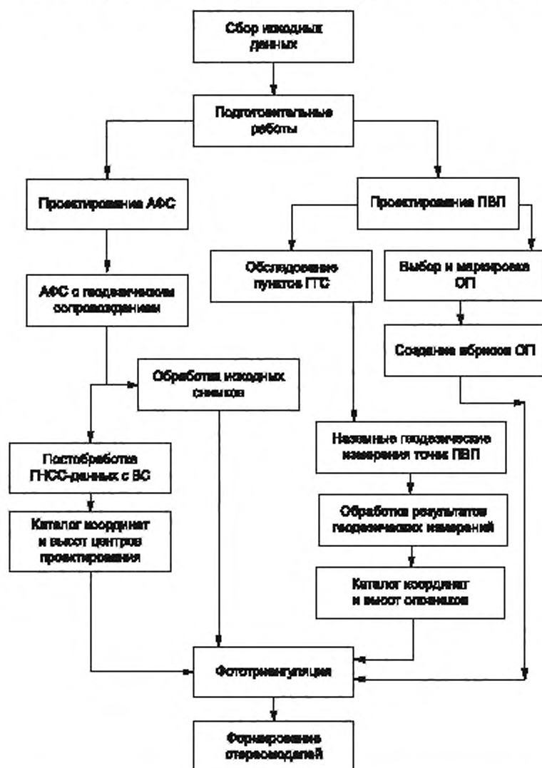
Рисунок А.1 — Технологическая схема создания ориентированных снимков для построения фотограмметрических стереомоделей местности
