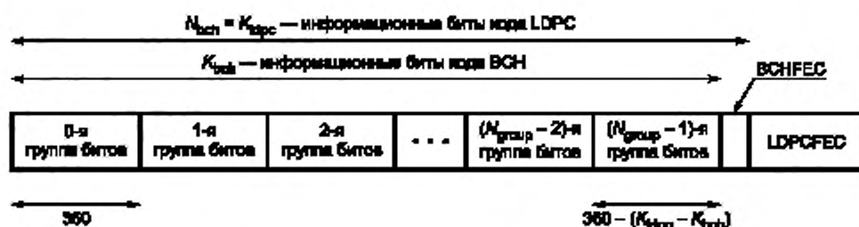
Рисунок 24 — Формат групп битов после LDPC-кодирования данных L1-сигнализации
