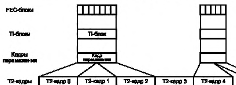
Рисунок 16 — Перемежение по времени для P_1 = 2 , I_{\text{JUMP}} = 2 , N_{T1} = 1
