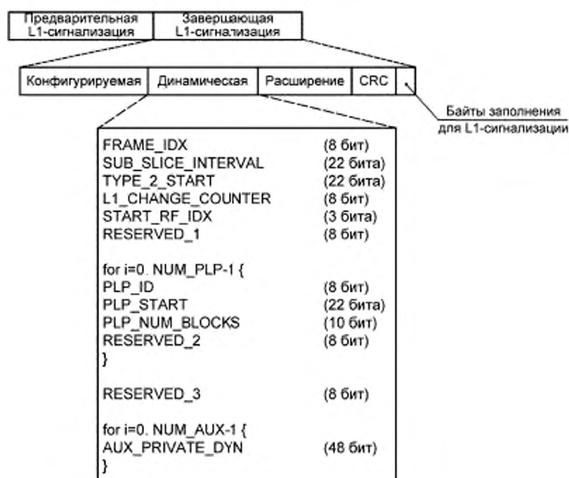
Рисунок 22 — Поля данных динамической завершающей L1-сигналикации
