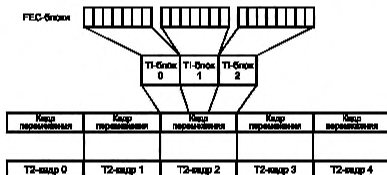
Рисунок 17 — Перемежение по времени для P_1 = 1 , I_{\text{JUMP}} = 1 , N_{T1} = 3
