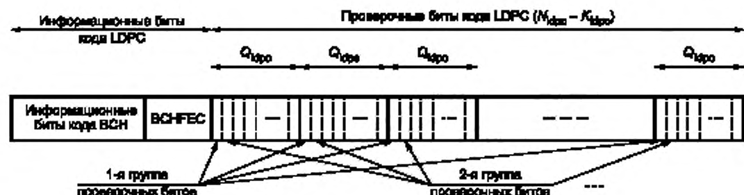
Рисунок 26 — Группы проверочных битов в FEC-блоке
