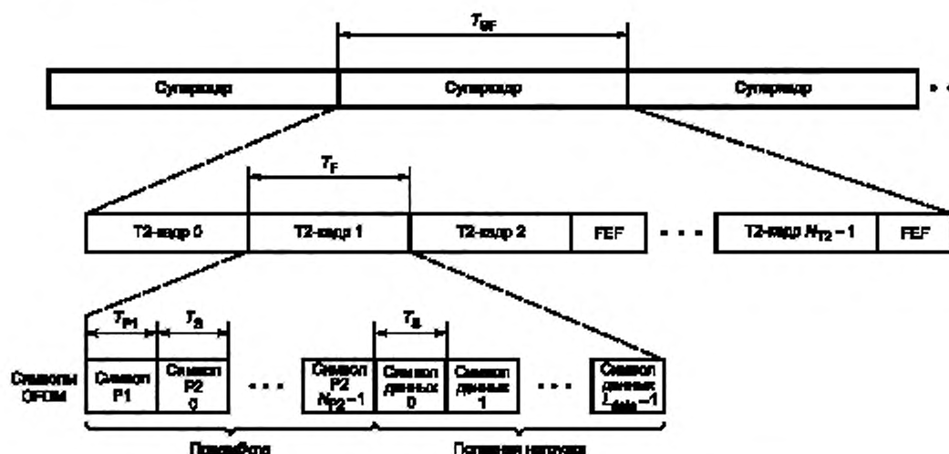
Рисунок 27 — Структура кадров системы DVB-T2 на физическом уровне
