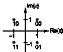
Рисунок 10 — Сигнальное созвездие при модуляции QPSK
