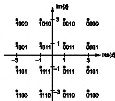
Рисунок 11 — Сигнальное созвездие при модуляции 16-QAM
