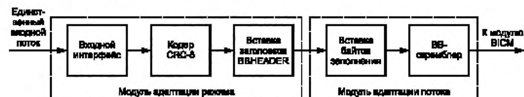
Рисунок 5 — Структурная схема модуля адаптации для режима ввода А
