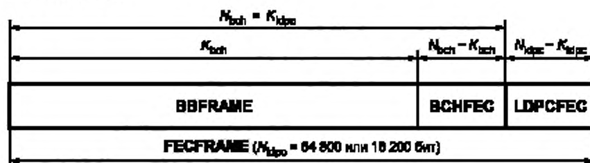
Рисунок 7 — Формат данных перед перемежением по битам
