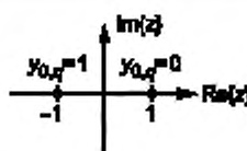
Рисунок 9 — Сигнальное созвездие при модуляции BPSK
