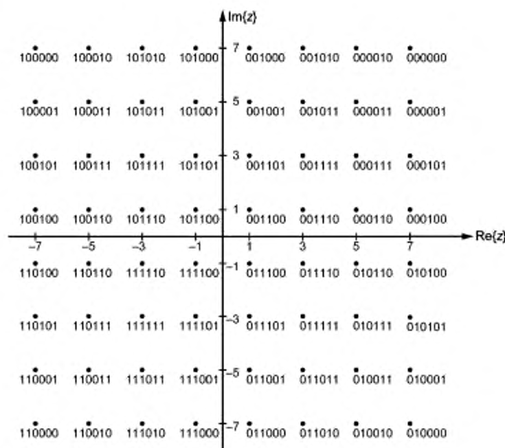
Рисунок 12 — Сигнальное созвездие при модуляции 64-QAM
