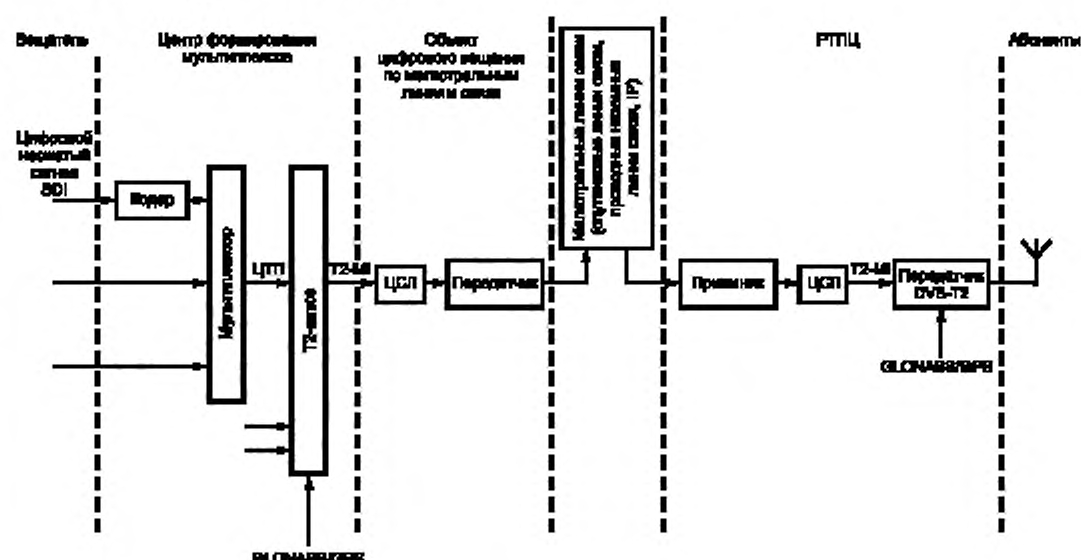
Рисунок 34 — Типовая структурная схема телевизионного вещания
