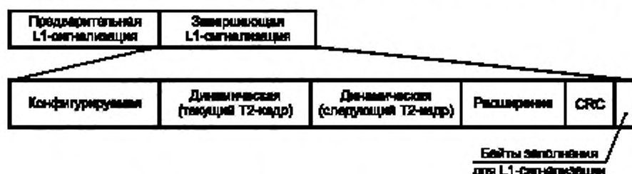
Рисунок 23 — Повторение информации динамической завершающей L1-сигналикации
