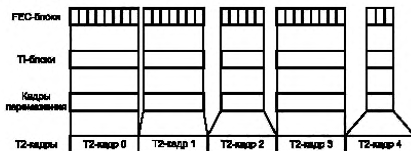
Рисунок 15 — Перемежение по времени для P_1 = 1 , I_{\text{JUMP}} = 1 , N_{T1} = 1
