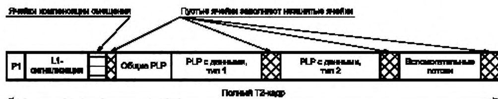
Рисунок 29 — Структура T2-кадра
