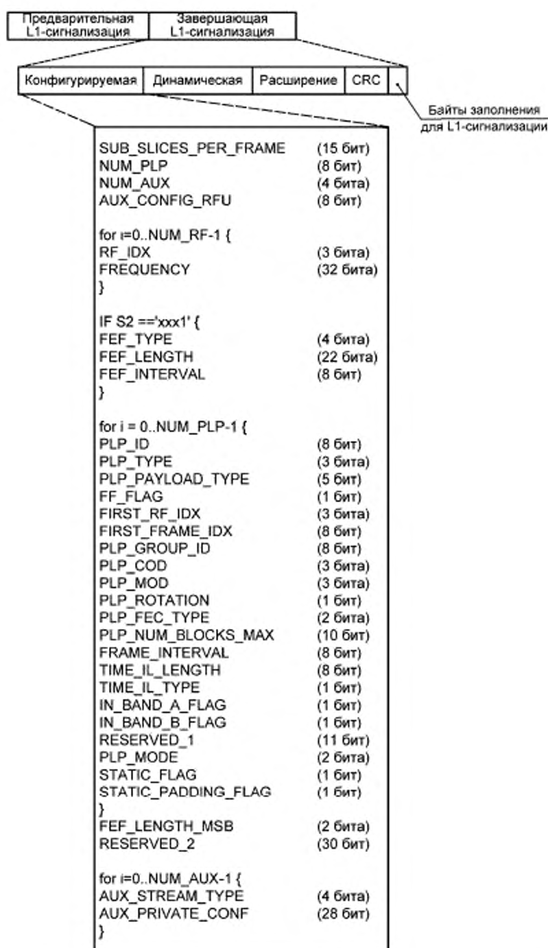
Рисунок 21 — Поля данных конфигурируемой завершающей L1-сигнализации
