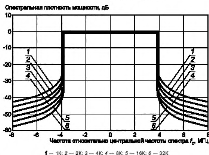
Рисунок 31 — Теоретический спектр сигнала OFDM
