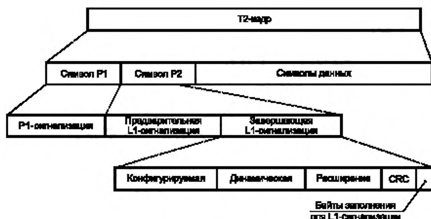
Рисунок 19 — Структура L1-сигнализации
