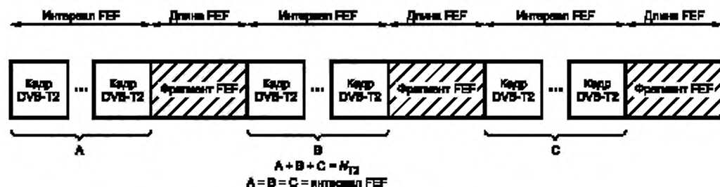
Рисунок 28 — Суперкадр, включающий T2-кадры и фрагменты FEF
