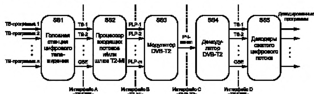
Рисунок 1 — Высокоуровневая архитектура системы DVB-T2
