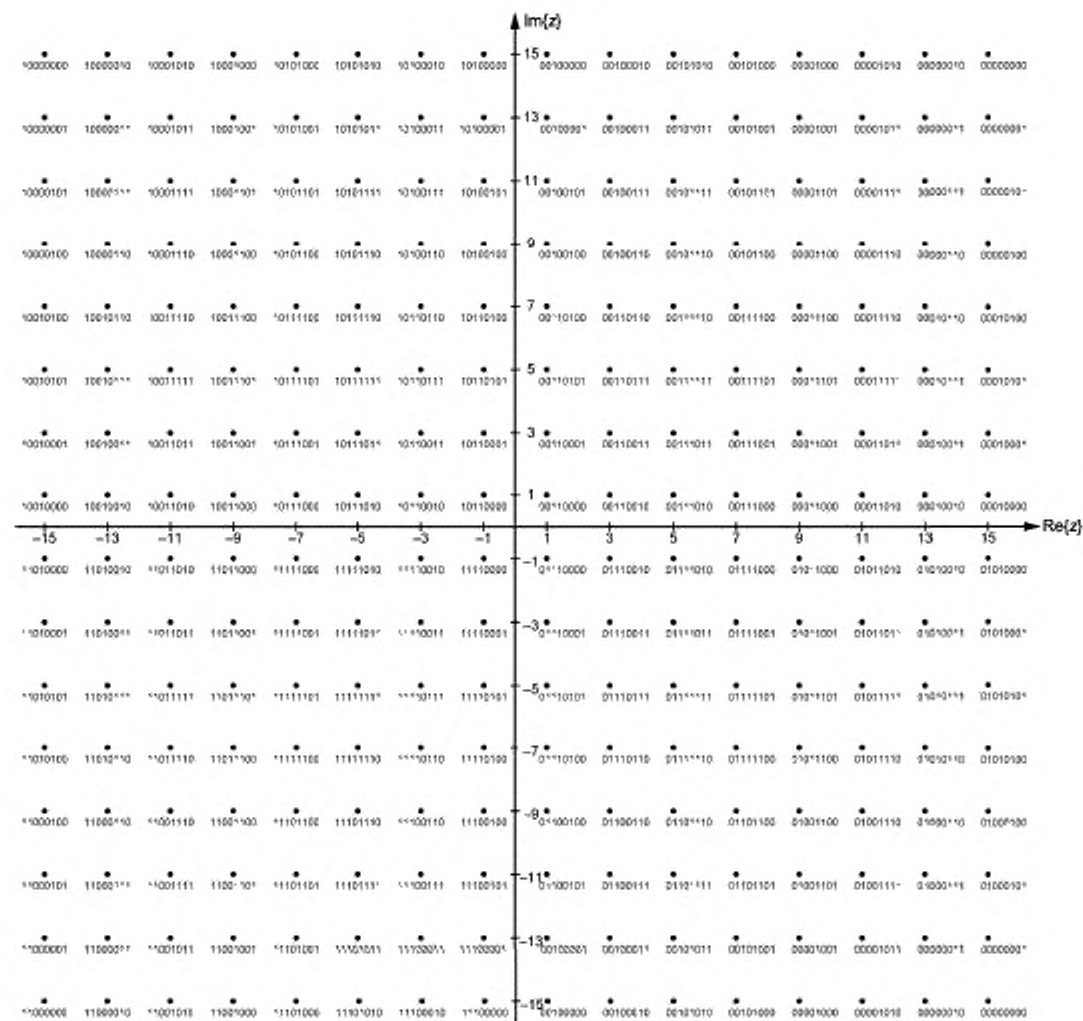
Рисунок 13 — Сигнальное созвездие при модуляции 256-QAM
