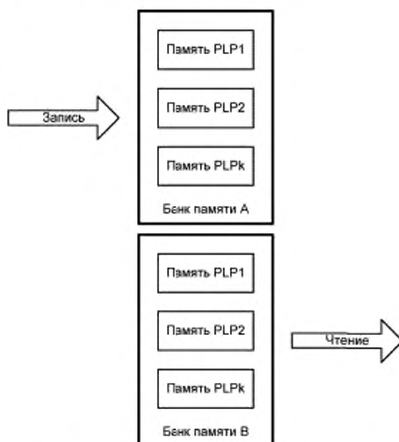
Рисунок 18 — Структура перемежителя по времени
